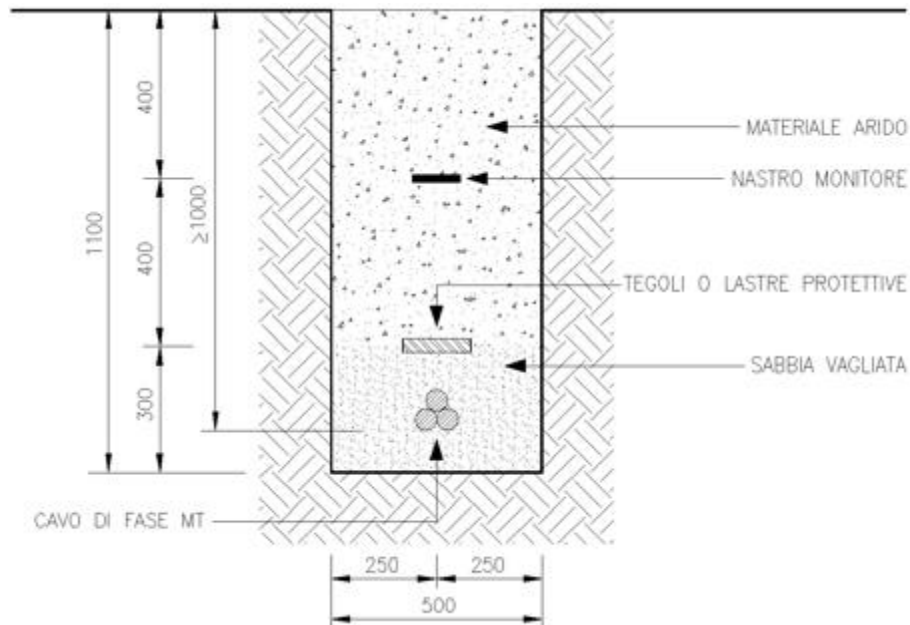
Tavola n. 13 Sezione tipica cavidotto interrato linea MT (n° 1 terna)
