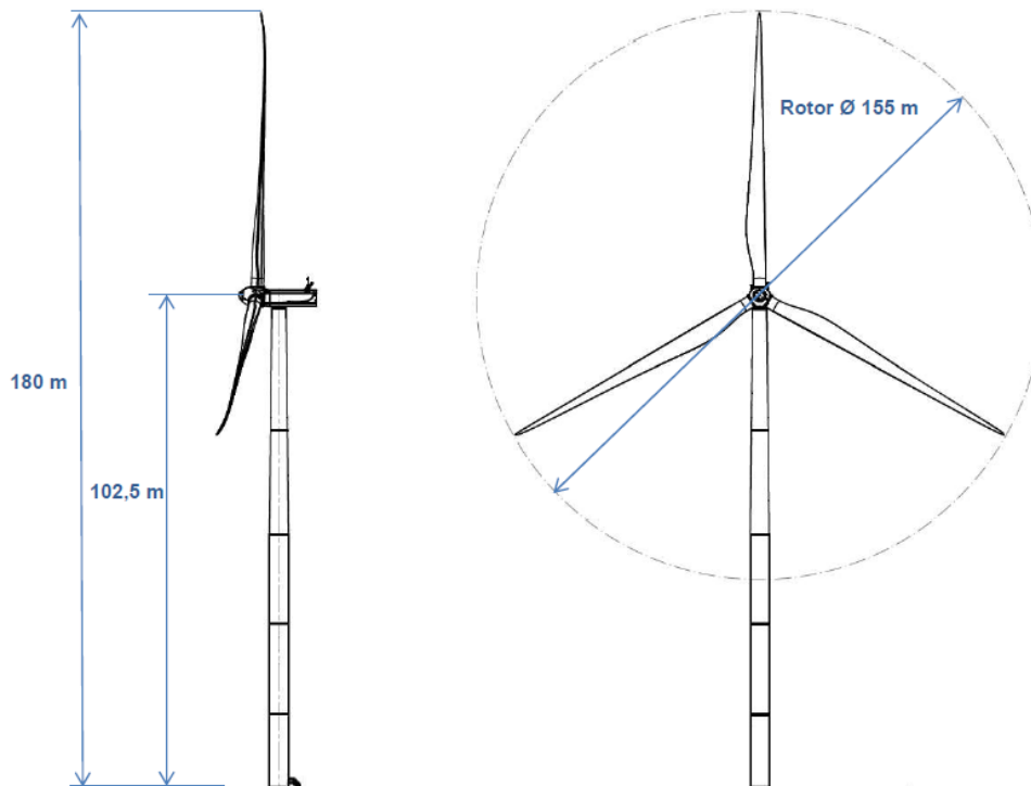
Figura 2 – Vista prospettica e laterale dell'aerogeneratore SIEMENS GAMESA SG 6.0 - 155 da 6,0 MW.
