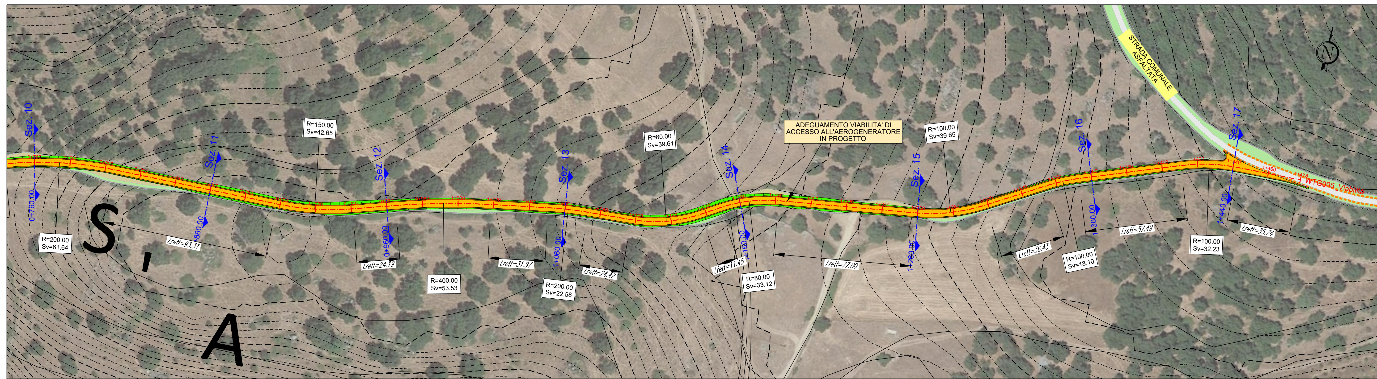
AEROGENERATORE WTG005 NUOVA VIABILITA' E ADEGUAMENTO DI QUELLA ESISTENTE - TAVOLA 2 Base carta: Ortofoto Google Map e C.T.R. Regione Sardegna
