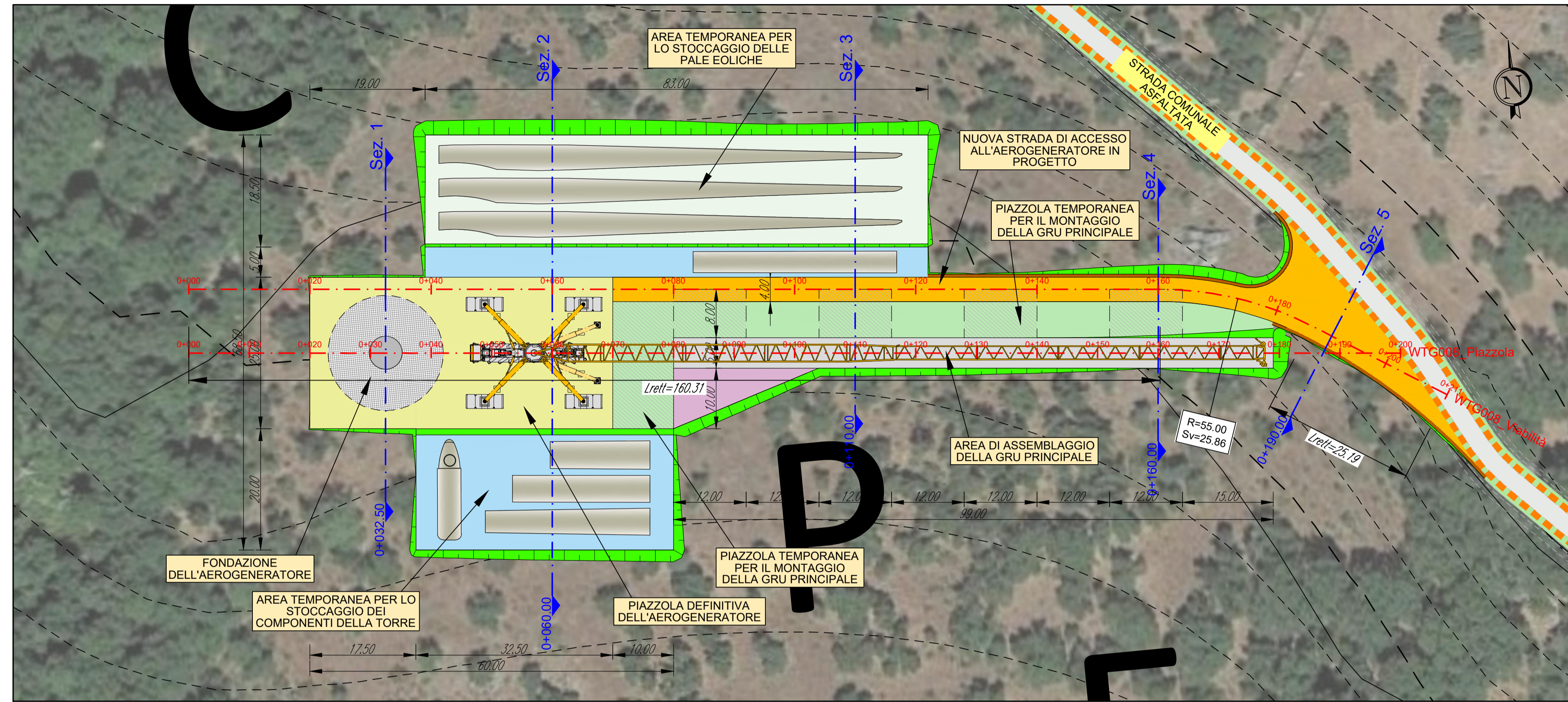
AEROGENERATORE WTG008 PIAZZOLA DI CANTIERE E NUOVA VIABILITA' DI ACCESSO Base carta: Ortofoto Google Map e C.T.R. Regione Sardegna Scala 1 : 500
