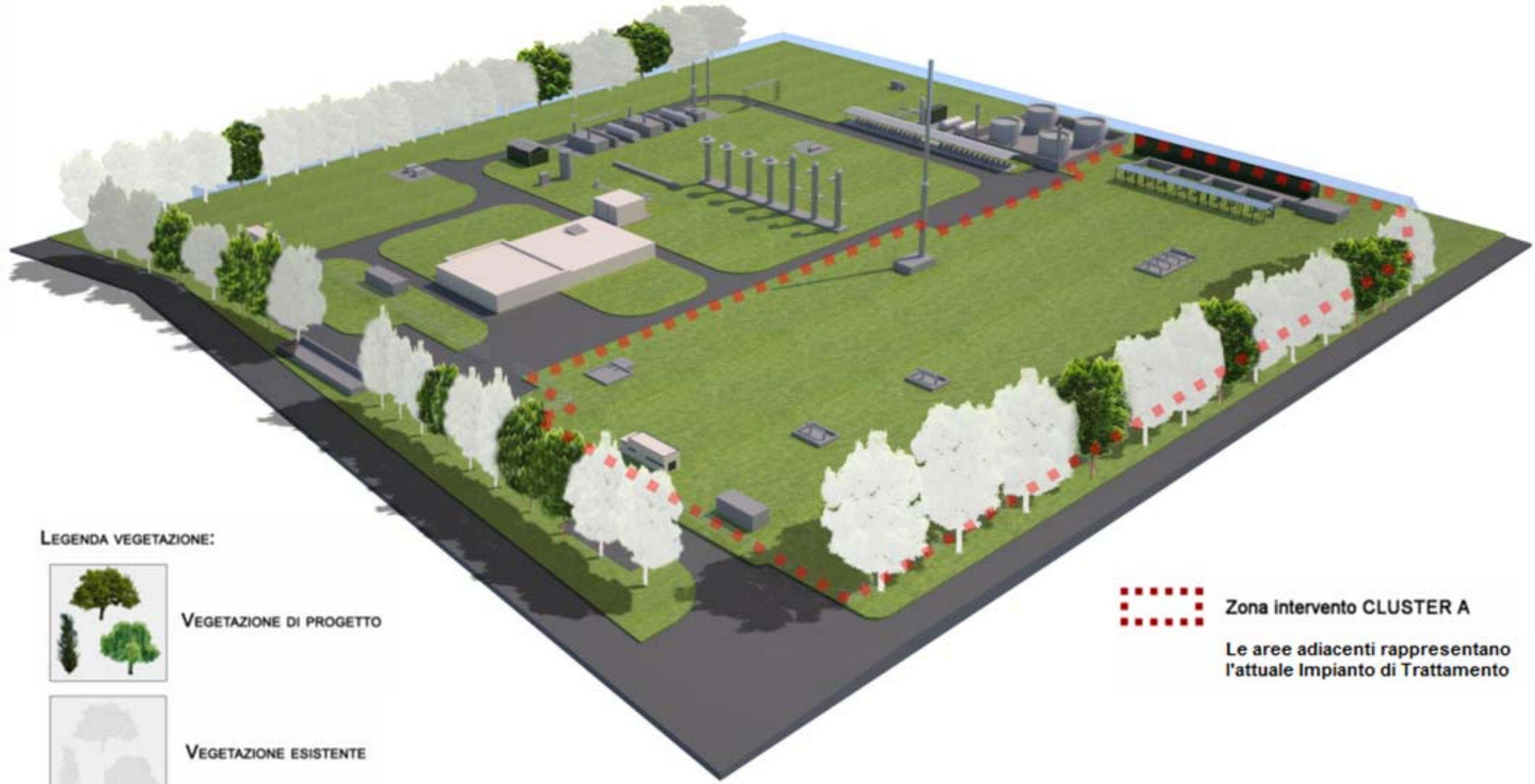
CENTRALE DI STOCCAGGIO GAS RIPALTA - CLUSTER A Fotosimulazione Impianto e Mitigazioni a verde - Vista 02
