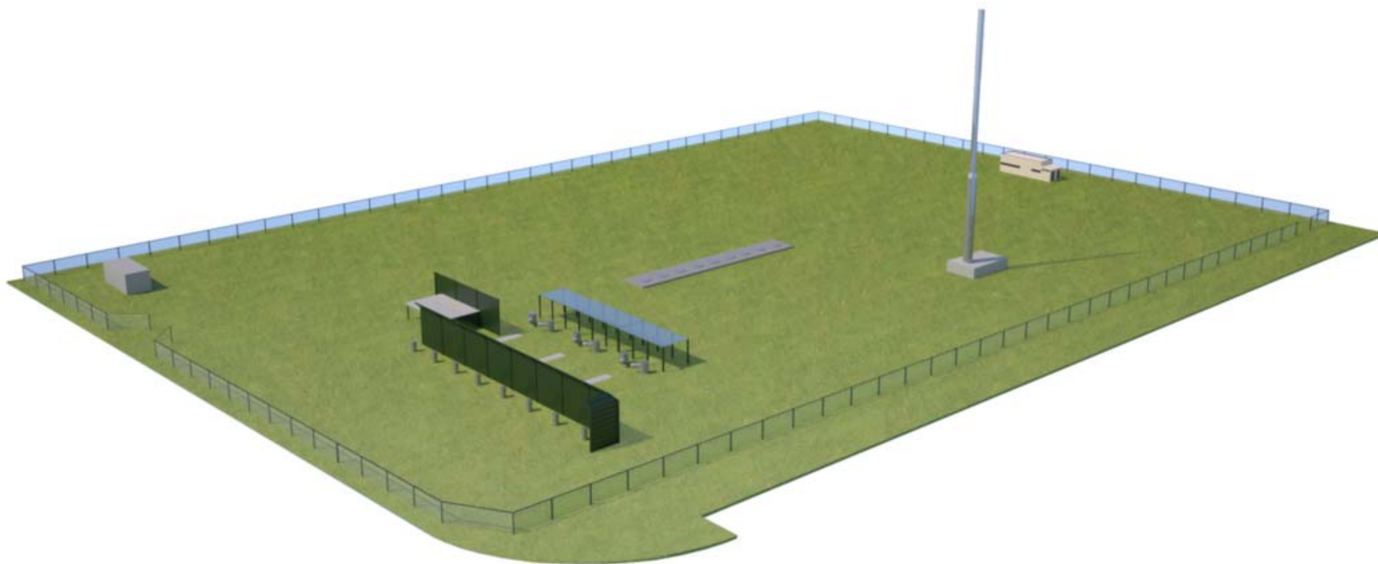
CENTRALE DI STOCCAGGIO GAS RIPALTA - CLUSTER D Fotosimulazione Impianto - Vista 01
