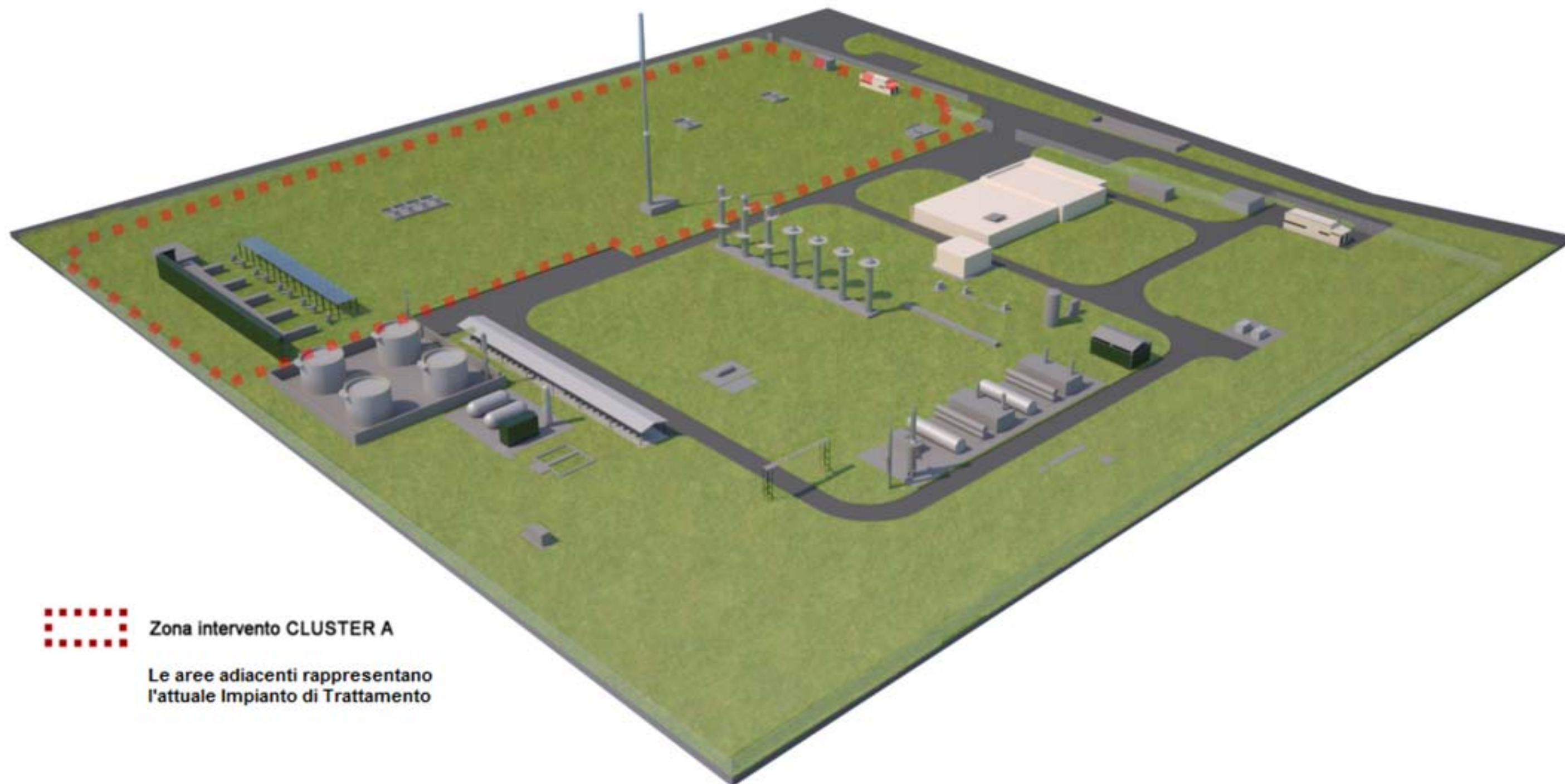
CENTRALE DI STOCCAGGIO GAS RIPALTA - CLUSTER A Fotosimulazione Impianto - Vista 01
