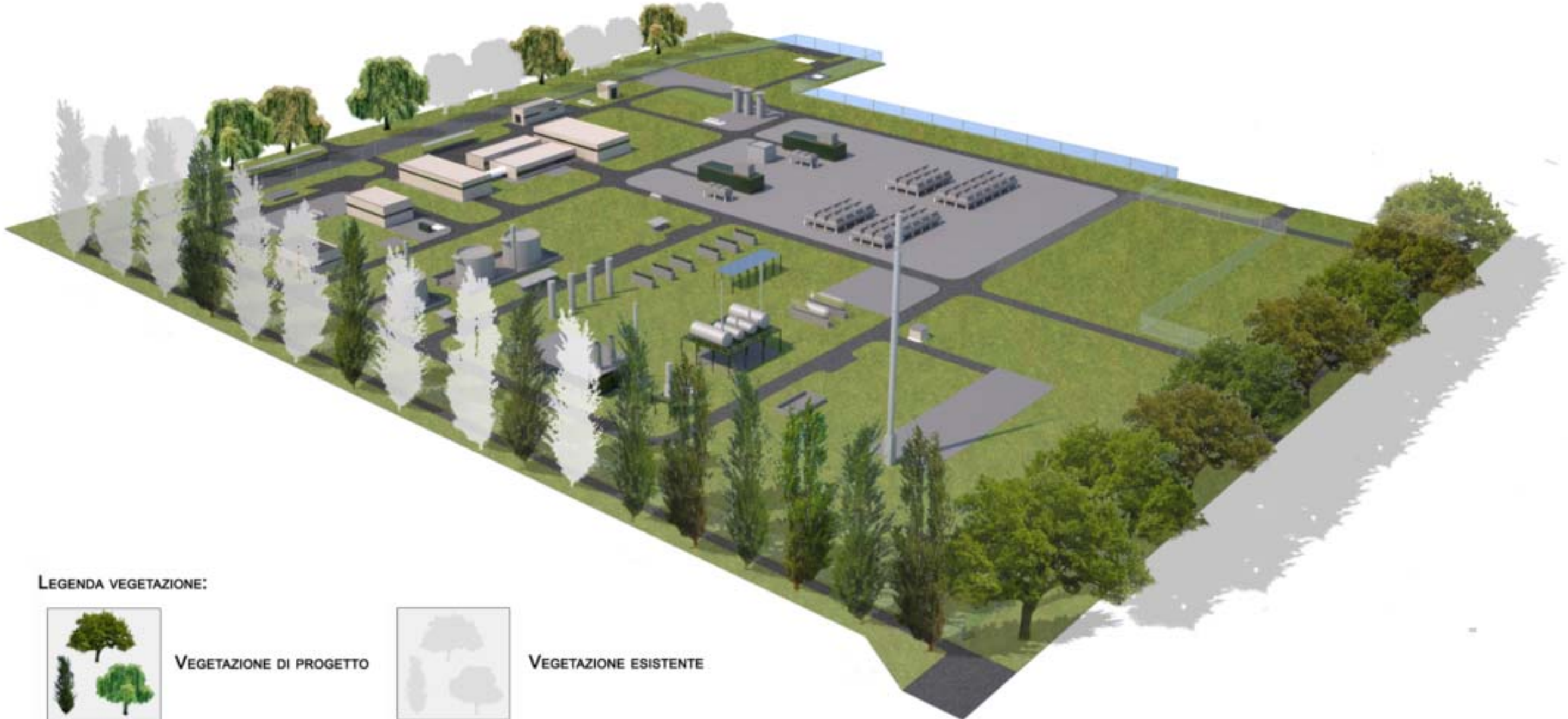
CENTRALE DI STOCCAGGIO GAS RIPALTA Fotosimulazione Impianto di trattamento gas e Mitigazione a verde - Vista 01
