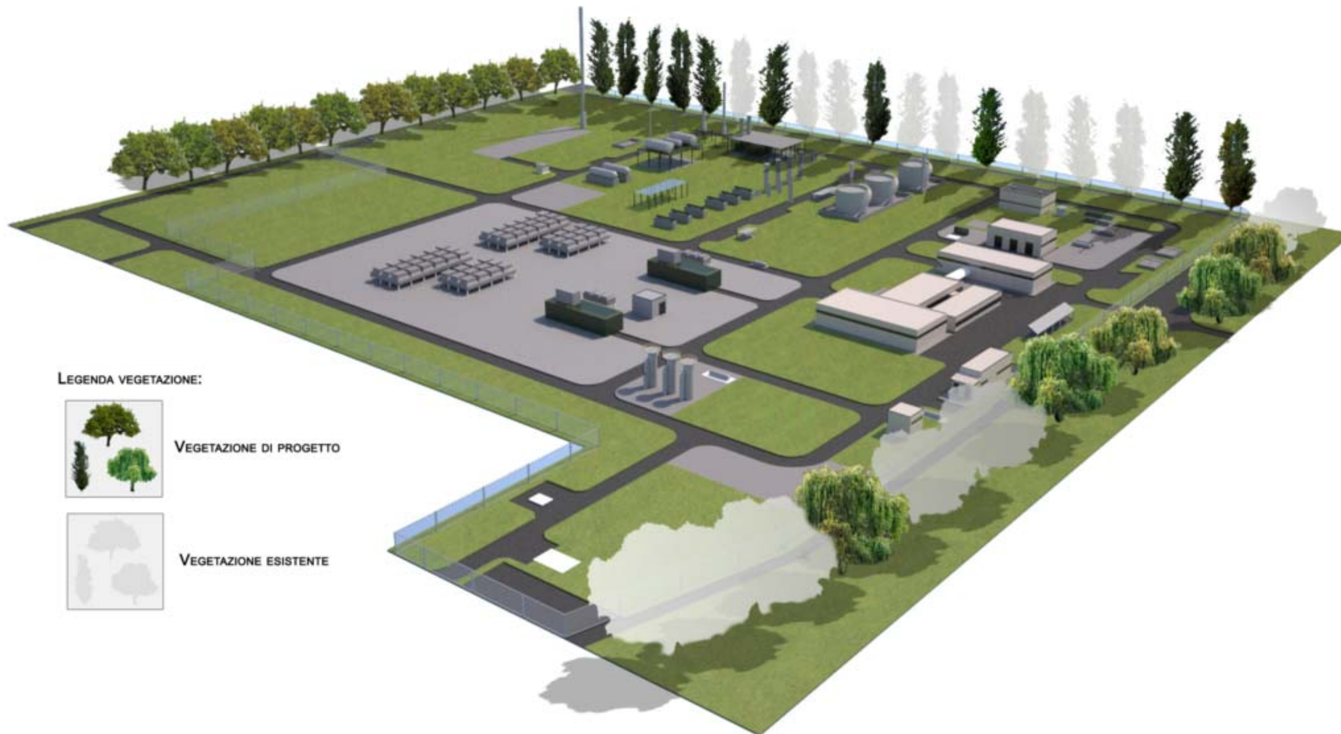
CENTRALE DI STOCCAGGIO GAS RIPALTA Fotosimulazione Impianto di trattamento gas e Mitigazione a verde - Vista 02
