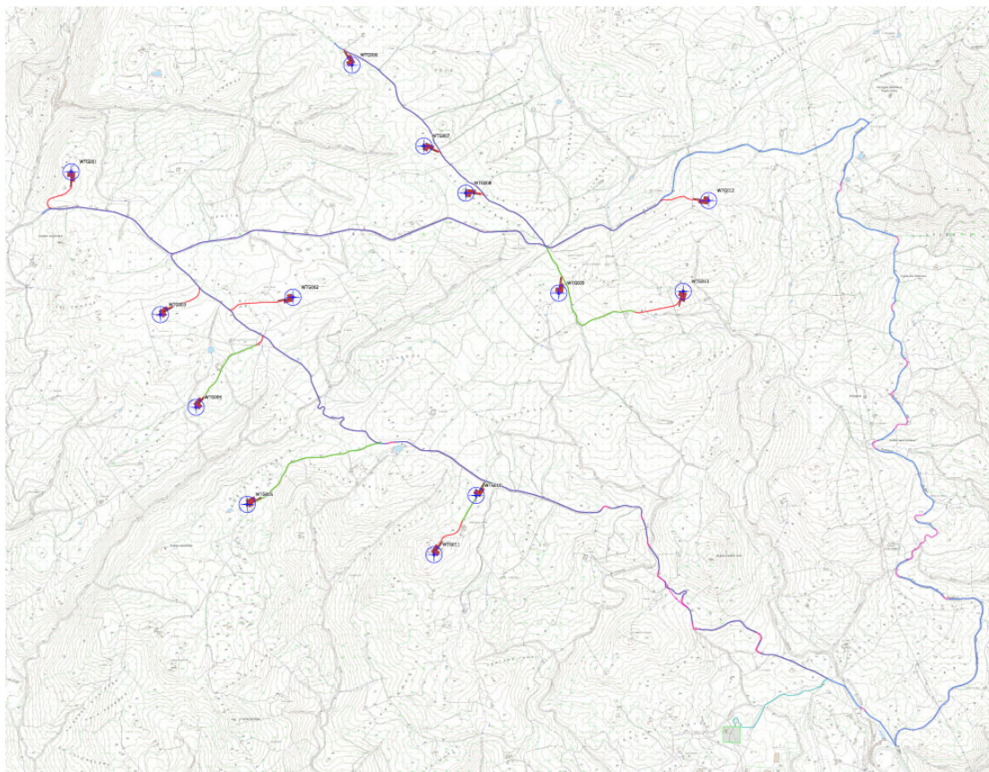
Figura 1 Layout progetto definitivo su base CTR
