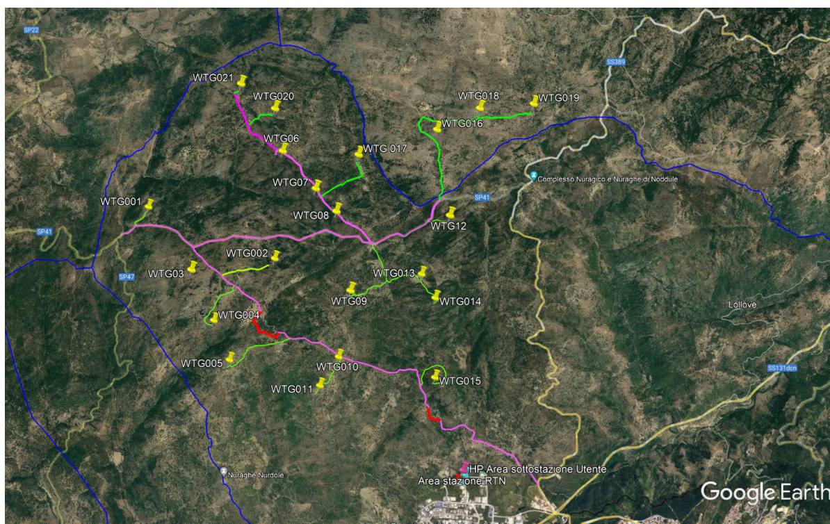
Figura 8 Layout dell'alternativa progettuale
