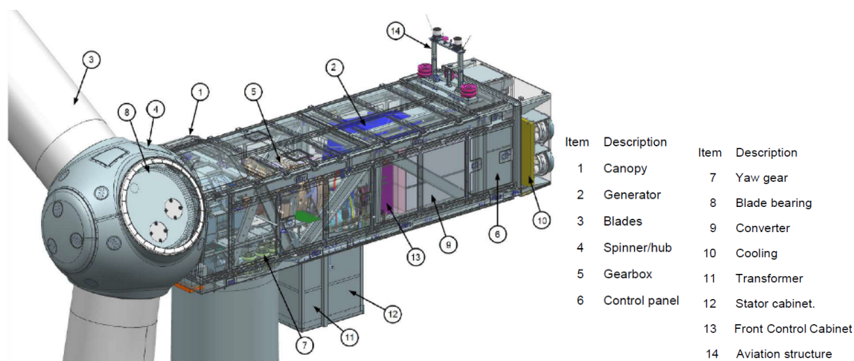
Figura 4 – Componenti dell'aerogeneratore
