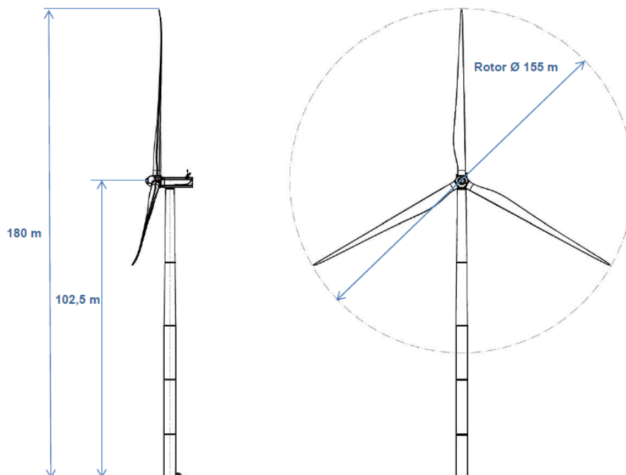
Figura 3 Schema geometrico degli aerogeneratori in progetto SG 6.0 - 155
