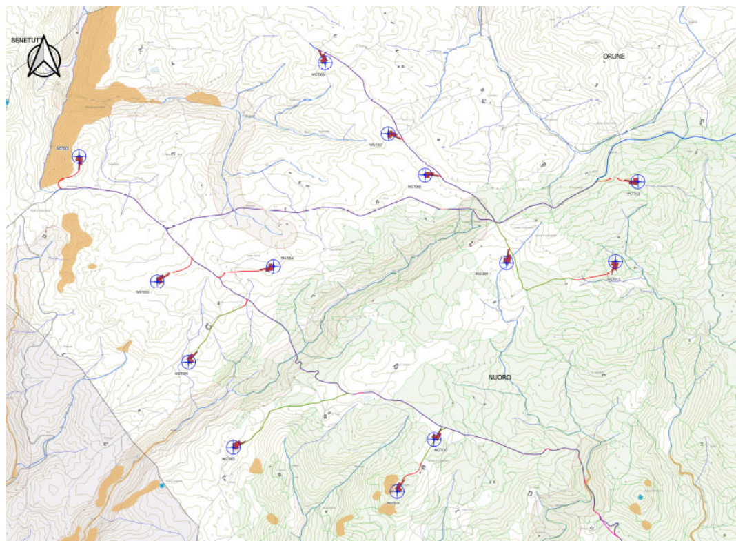
Figura 6 Stralcio cartografia elaborato V.2.5. Aree non idonee impianti FER
