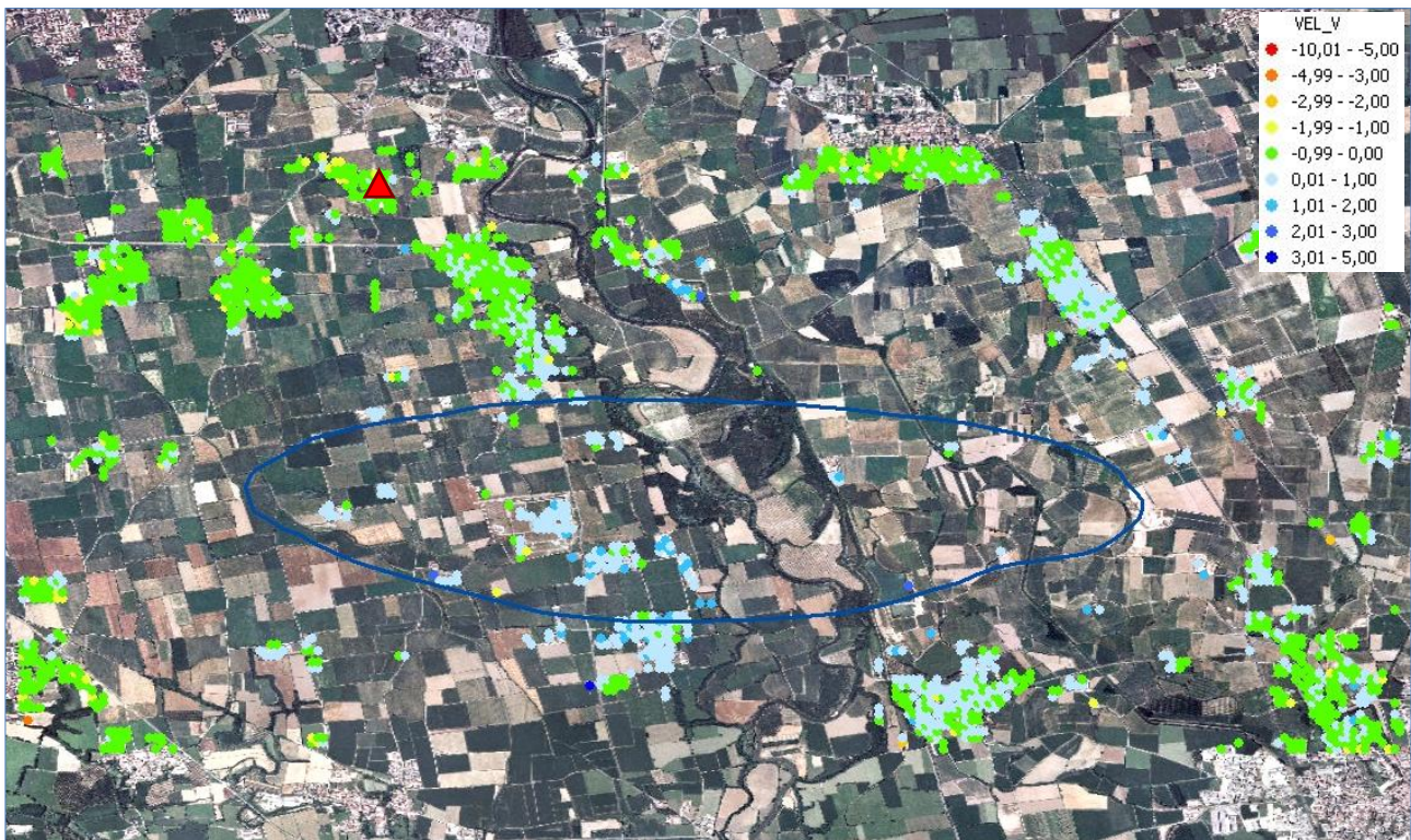
Fig.12 Visualizzazione in scala di colori delle velocità verticali dei punti scomposti del rilievo LOCAL, così come registrati originariamente dal satellite.
