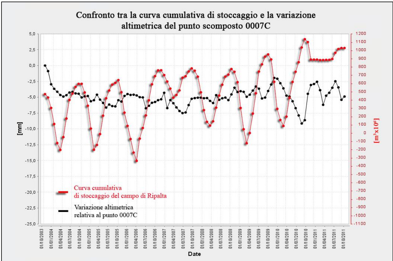
Fig.21 Confronto tra l'andamento temporale delle variazioni altimetriche del punto scomposto 0007C e la curva cumulativa di stoccaggio del giacimento di Ripalta.
