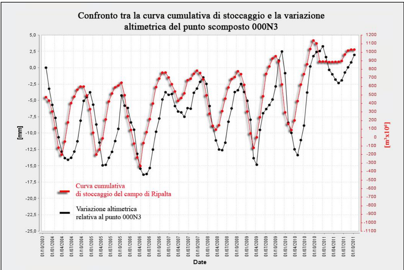
Fig.19 Confronto tra l'andamento temporale delle variazioni altimetriche del punto scomposto 000N3 e la curva cumulativa di stoccaggio del giacimento di Ripalta.
