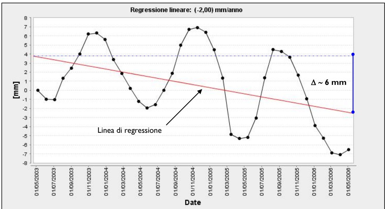
Fig.15 Esempio di serie storica con valori di subsidenza di circa 2 mm/anno.
