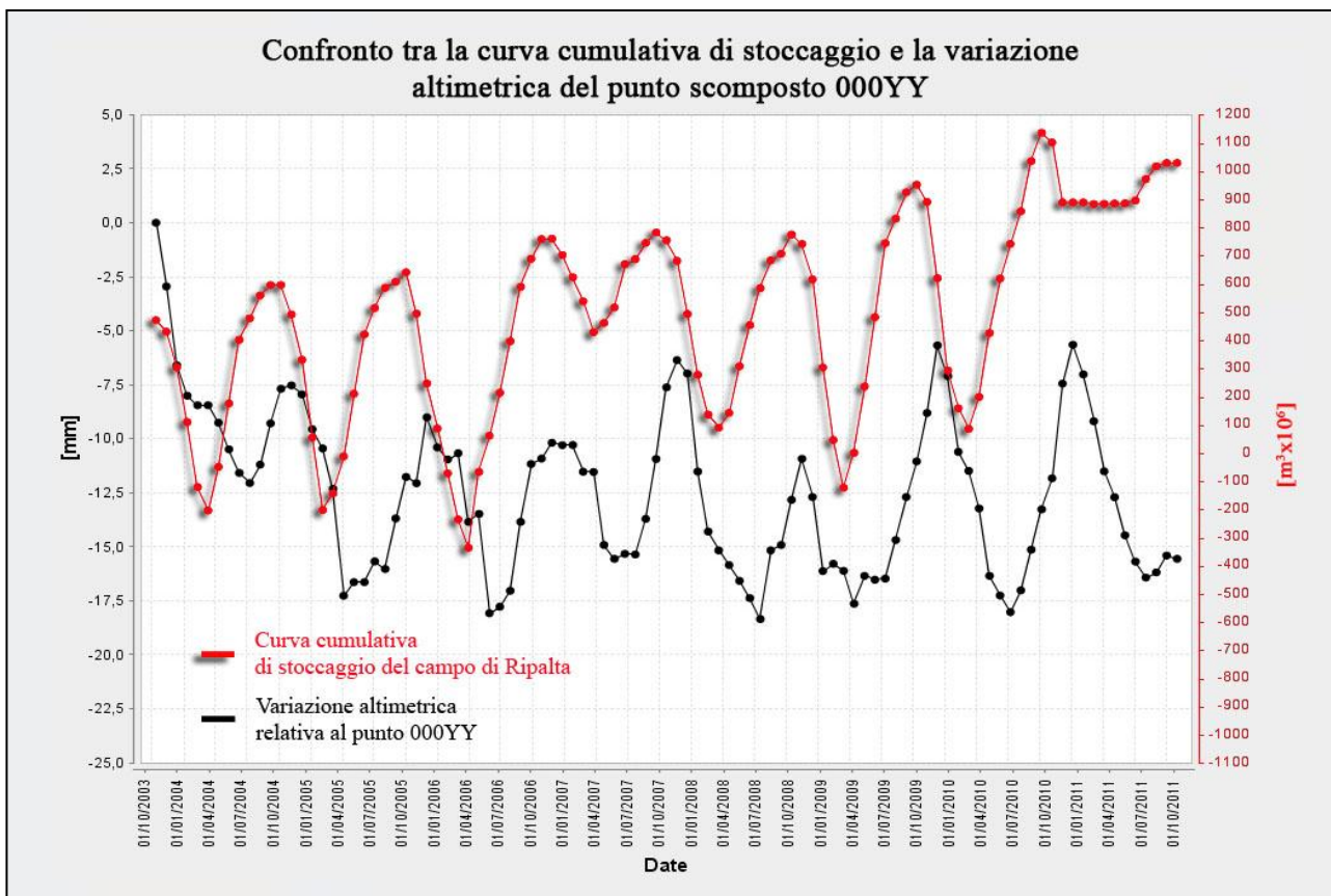
Fig.20 Confronto tra l'andamento temporale delle variazioni altimetriche del punto scomposto 000YY e la curva cumulativa di stoccaggio del giacimento di Ripalta.
