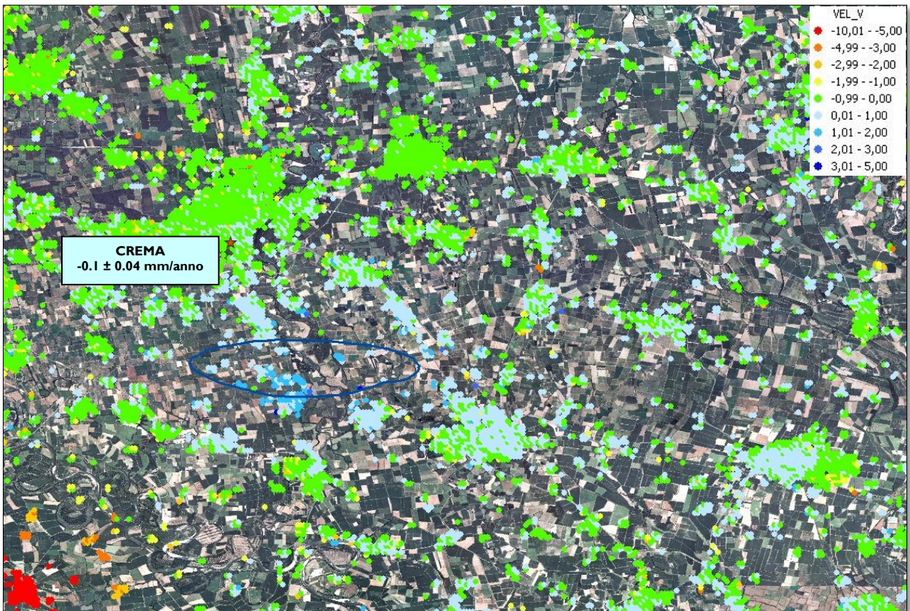
Fig.9 Dettaglio dei valori di velocità verticali sull'area del giacimento di stoccaggio di Ripalta.
