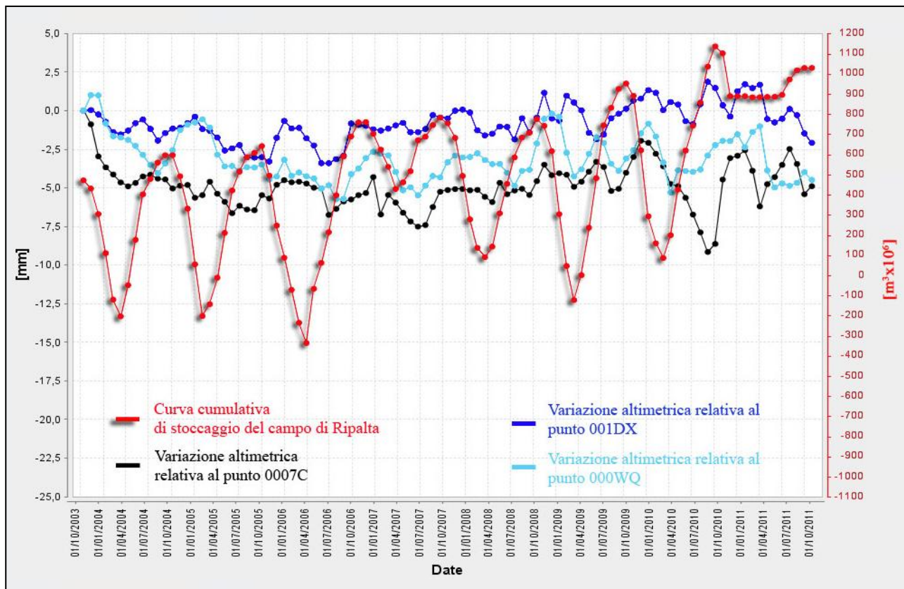
Fig.25 Confronto tra la curva cumulativa di stoccaggio del giacimento di Ripalta e le serie storiche dei punti scelti all'esterno dei limiti del campo.
