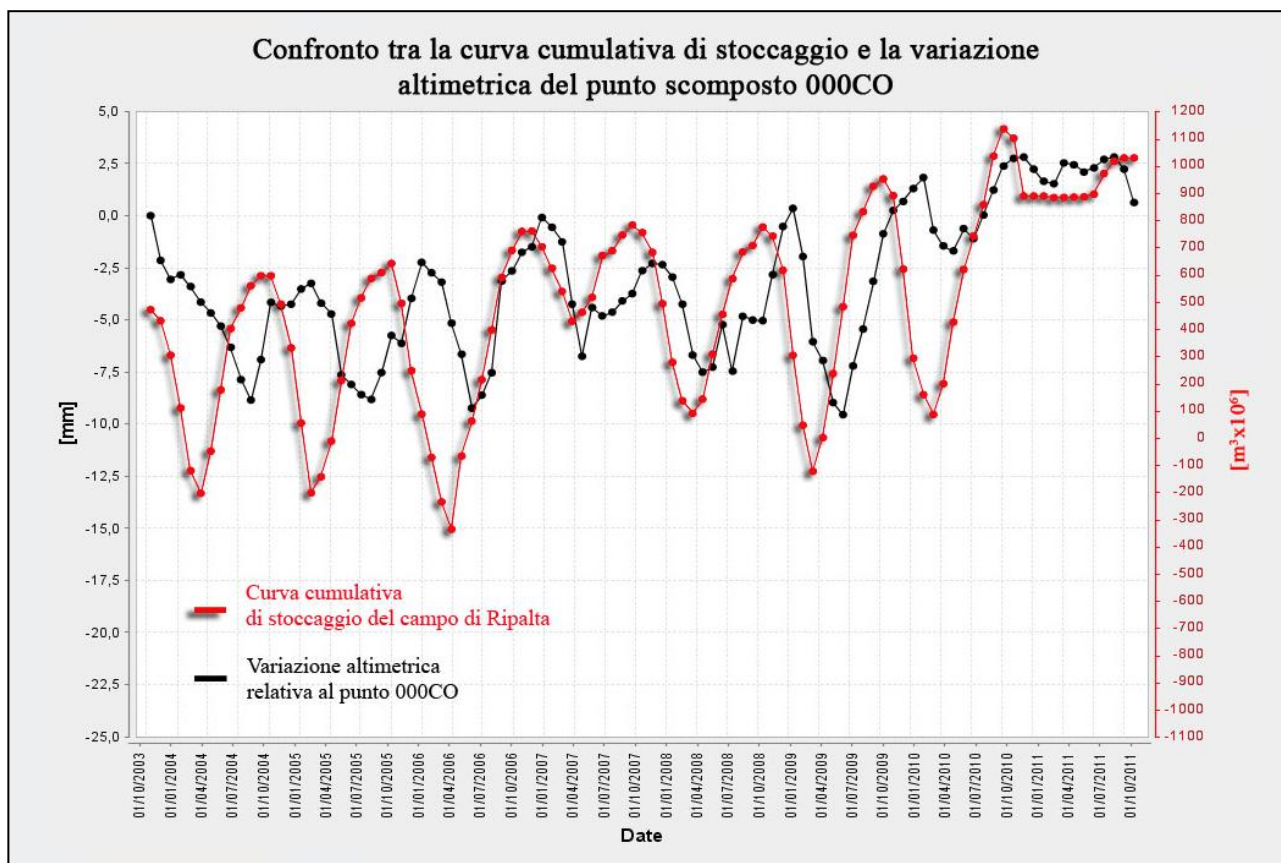
Fig.18 Confronto tra l'andamento temporale delle variazioni altimetriche del punto scomposto 000CO e la curva cumulativa di stoccaggio del giacimento di Ripalta.
