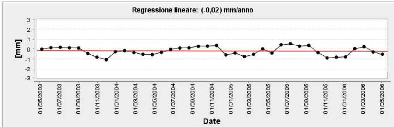
Fig.16 Esempio di serie storica con valori di regressione lineare nulla.
