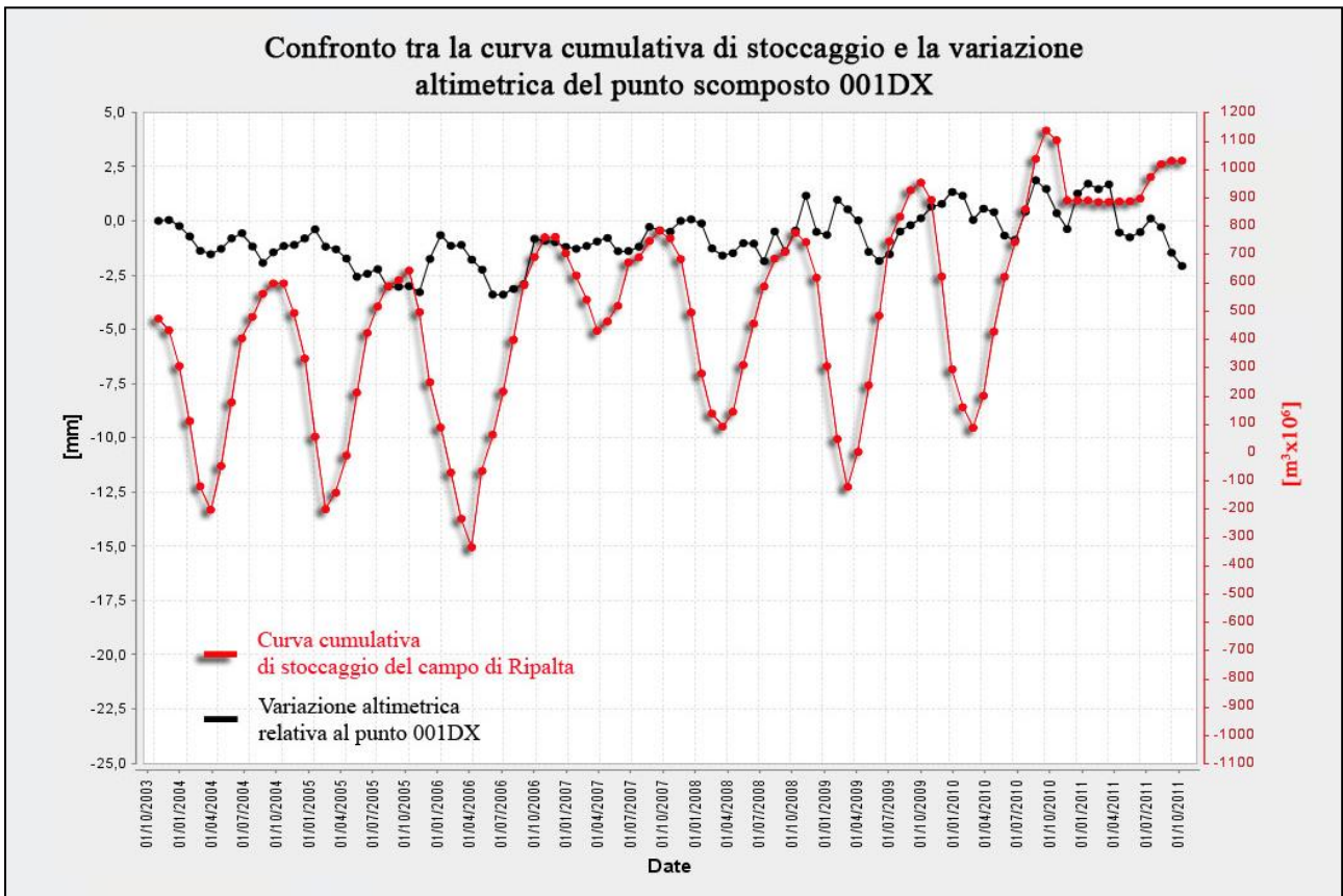
Fig.23 Confronto tra l'andamento temporale delle variazioni altimetriche del punto scomposto 001DX e la curva cumulativa di stoccaggio del giacimento di Ripalta.
