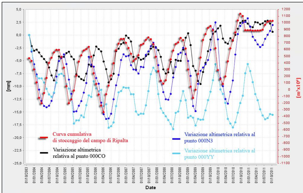
Fig.24 Confronto tra la curva cumulativa di stoccaggio del giacimento di Ripalta e le serie storiche dei punti scelti all'interno dei limiti del campo.
