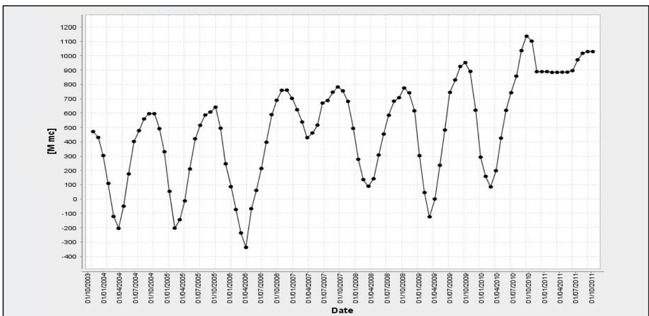
Fig.17 Curva cumulativa di stoccaggio del campo a gas di Ripalta (unità di misura in m^3 \times 10^6 ).
