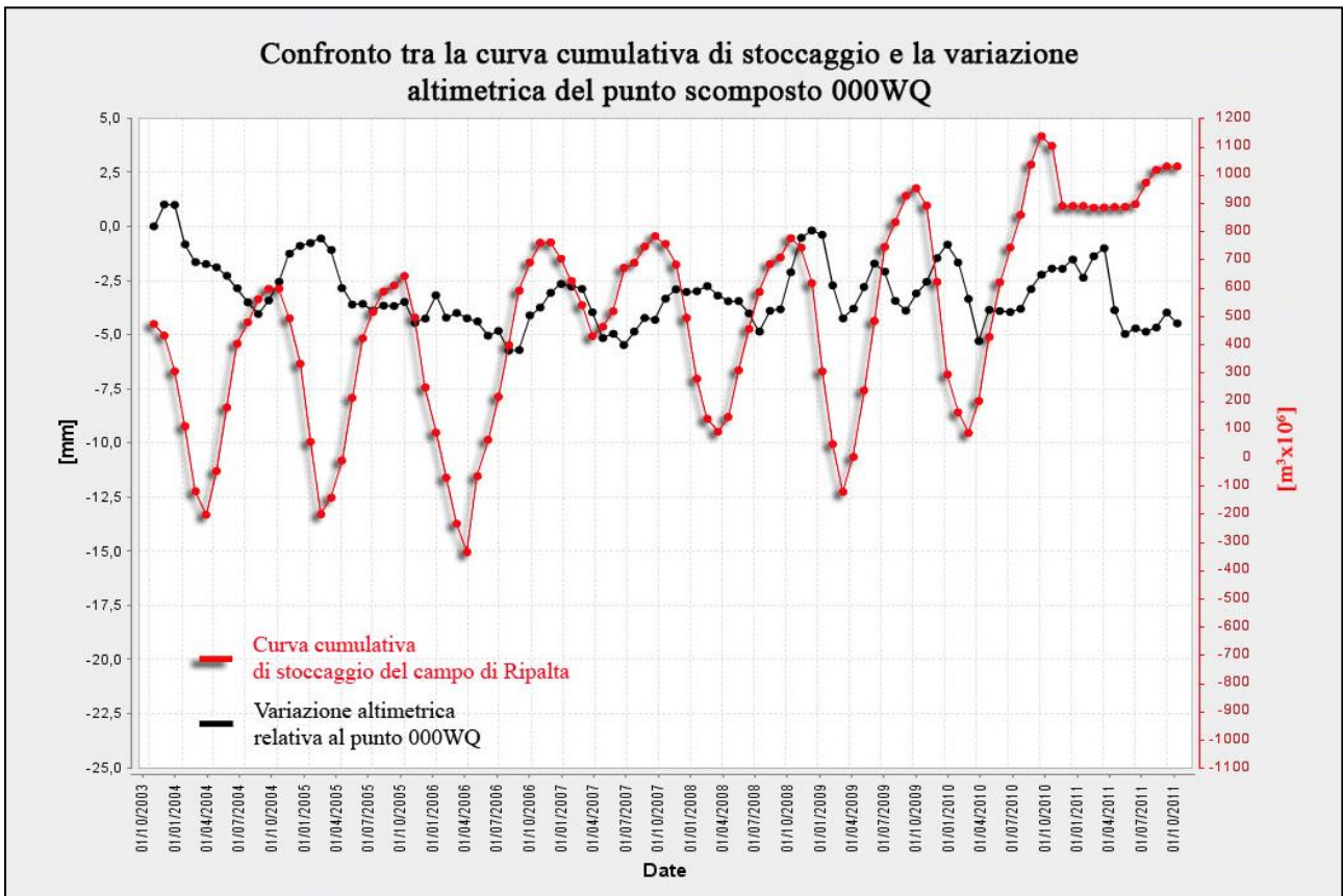
Fig.22 Confronto tra l'andamento temporale delle variazioni altimetriche del punto scomposto 000WQ e la curva cumulativa di stoccaggio del giacimento di Ripalta.
