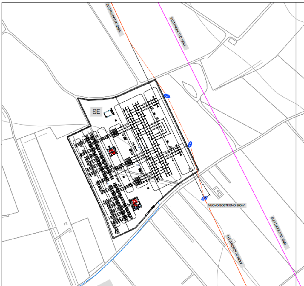
Figura 2: Layout Stazione elettrica
