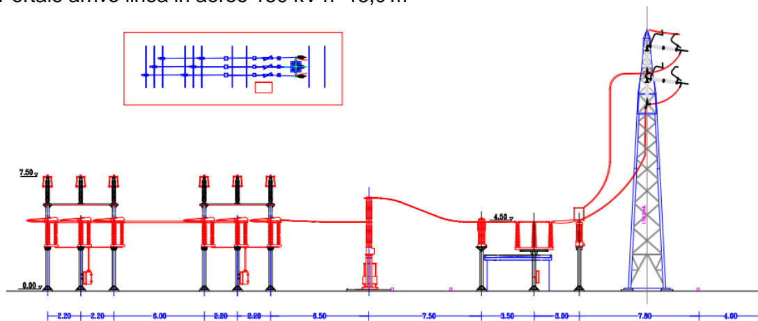
Prospetto stallo arrivo aereo a 150 kV
