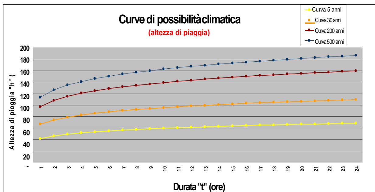
Figura 5. Curve di possibilità pluviometrica in funzione del tempo di ritorno (Tr) dell'evento (10, 30, 50, 100, 200 anni).
