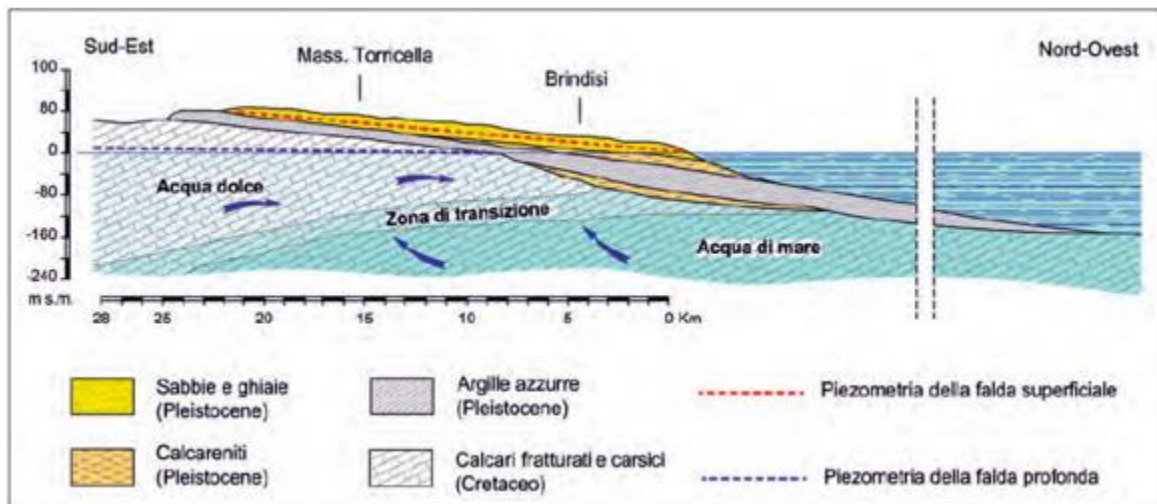
Tavola n. 16 - Schema idrico del territorio di Brindisi.
