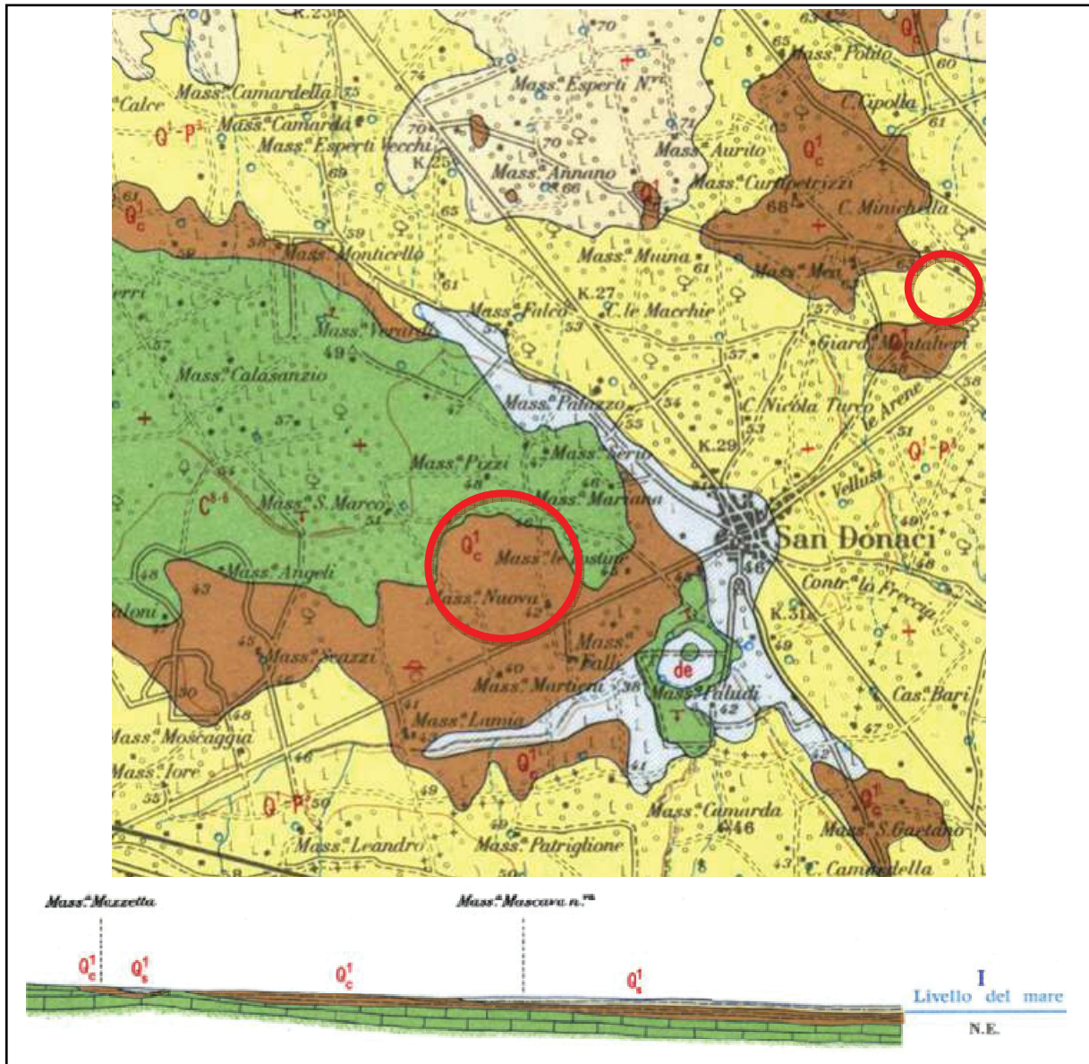
STRALCIO CARTA GEOLOGICA ISPRA – FOGLIO 203 BRINDISI
