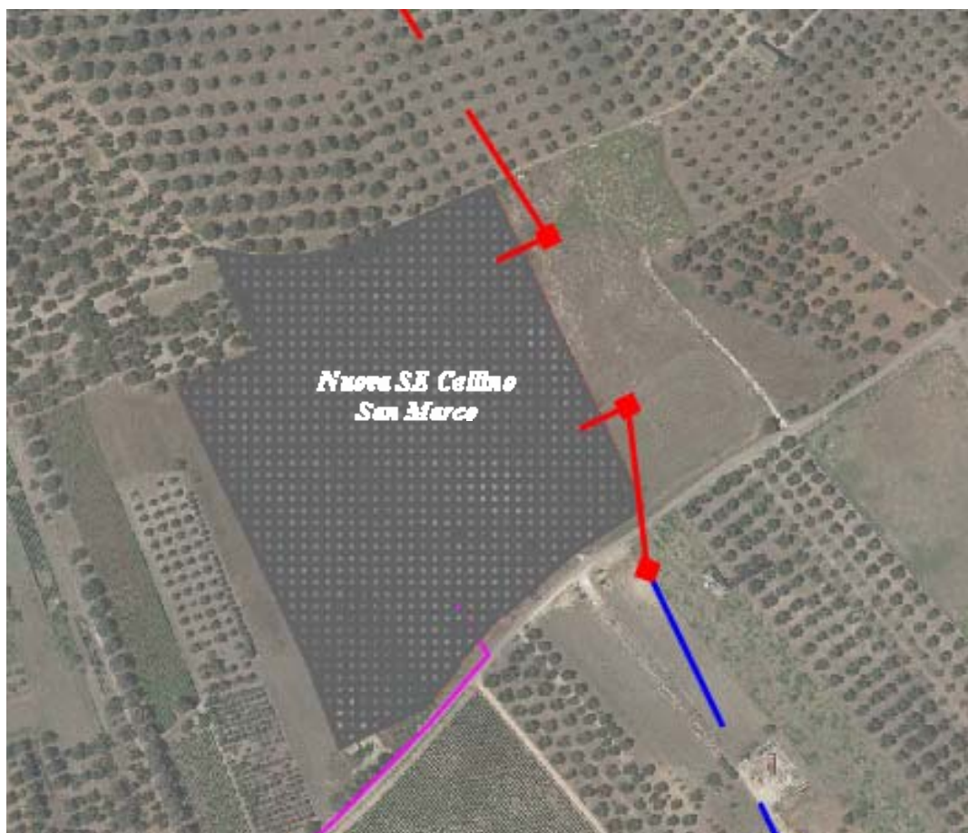
Stazione Elettrica Terna 380/150 kV "Cellino San Marco"
