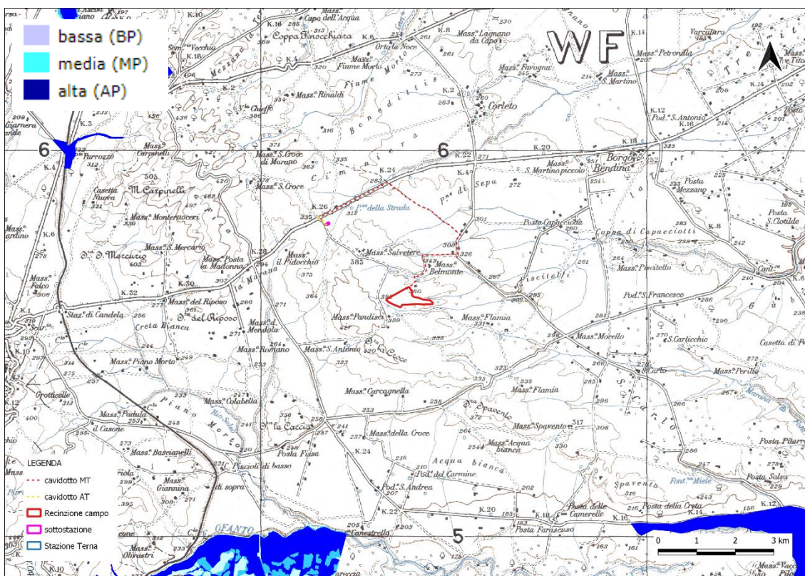
Figura 3 - Stralcio Carta Idrogeomorfologica del P.A.I.
