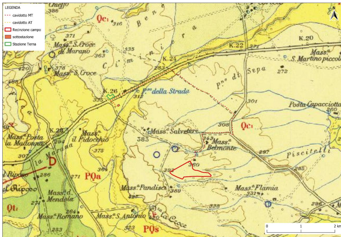
Figura 2 - Stralcio della carta geologica d'Italia fg.175 (Ascoli Satriano)
