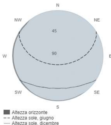
Figura 9 – Grafico dell'orizzonte
