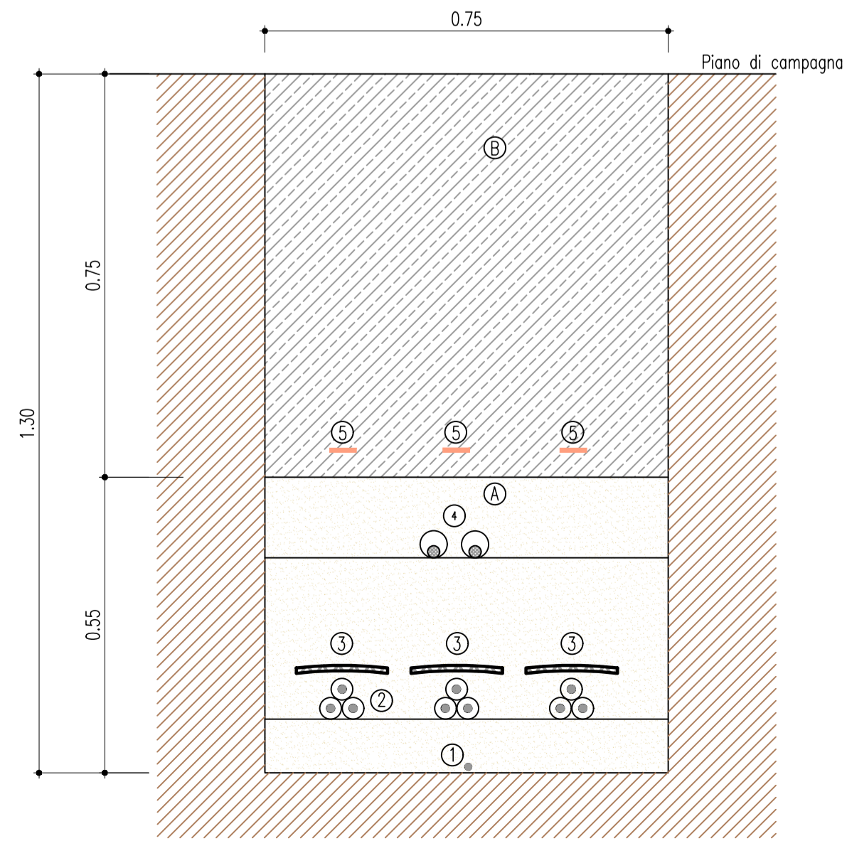
SEZIONE TIPO 3A - SU TERRENO IN FREGIO ALLA VIABILITA'
