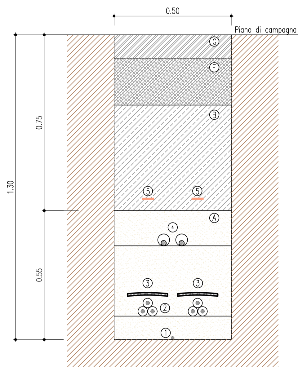
SEZIONE TIPO 2B - SU STRADA MISTATA
