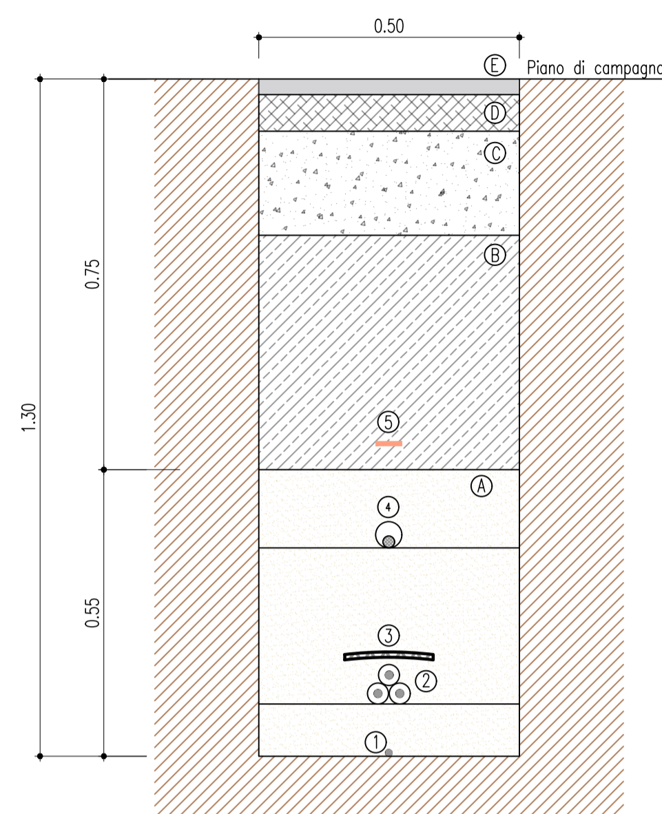
SEZIONE TIPO 2C - SU STRADA ASFALTATA
