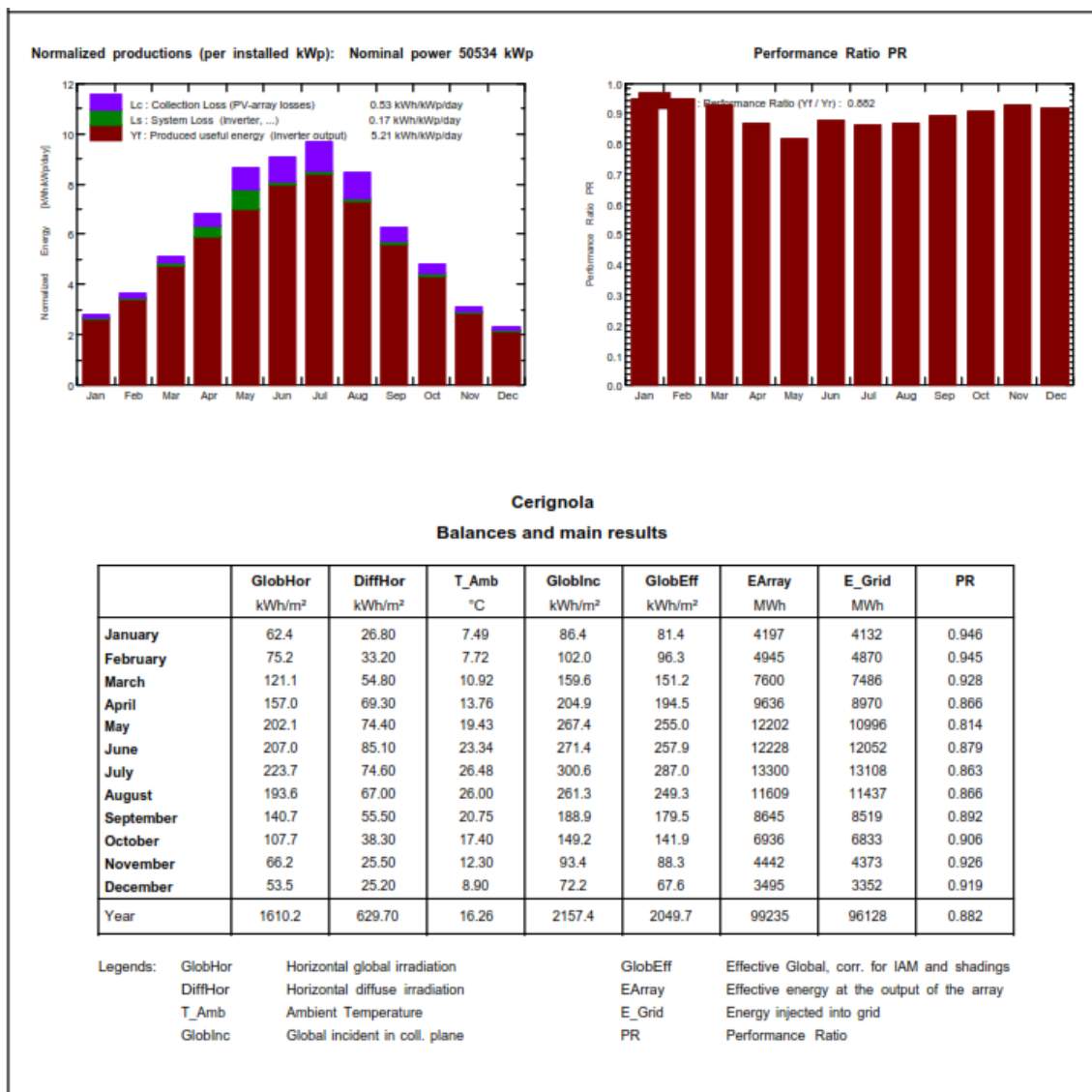
Figura 29; stralcio PVSyst
