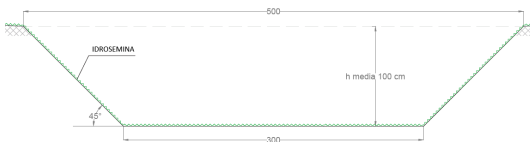
SEZIONE TIPO CANALE INTERNO A SUD-EST DELL'AREA D'IMPIANTO - scala 1:20
