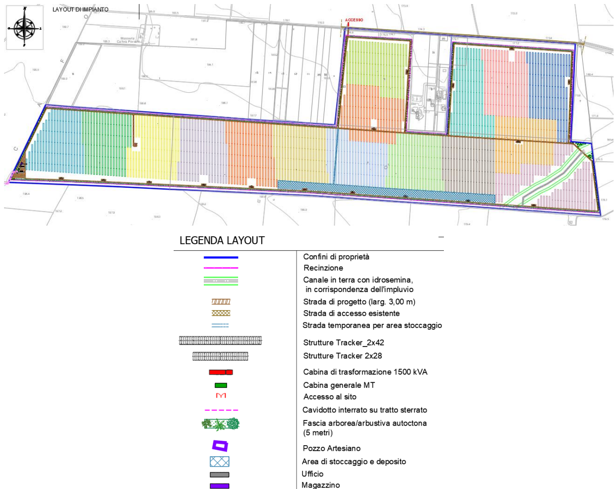
Figura 13 – Layout di progetto
