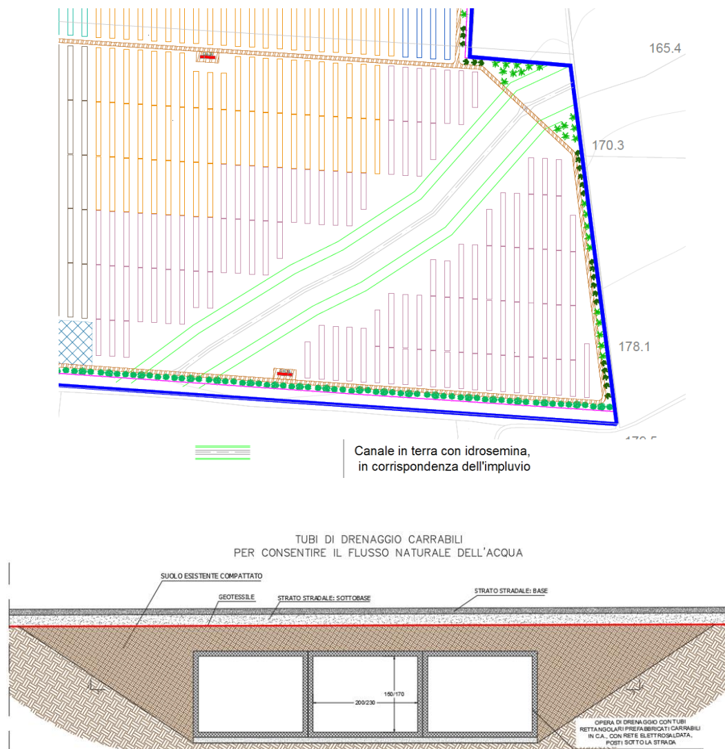
Figura 28 Porzione sud-est dell'area d'impianto in planimetria ed attraversamento tipo, sotto le strade: sia per la strada a nord che per quella a sud
