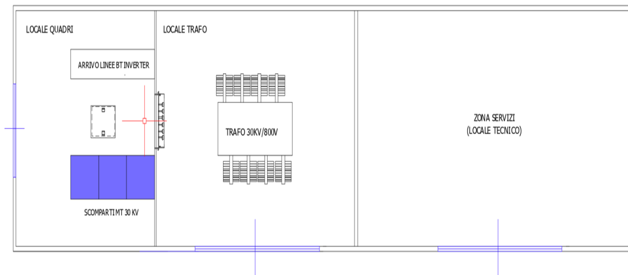
Figura 11 - Pianta cabina sottocampo
