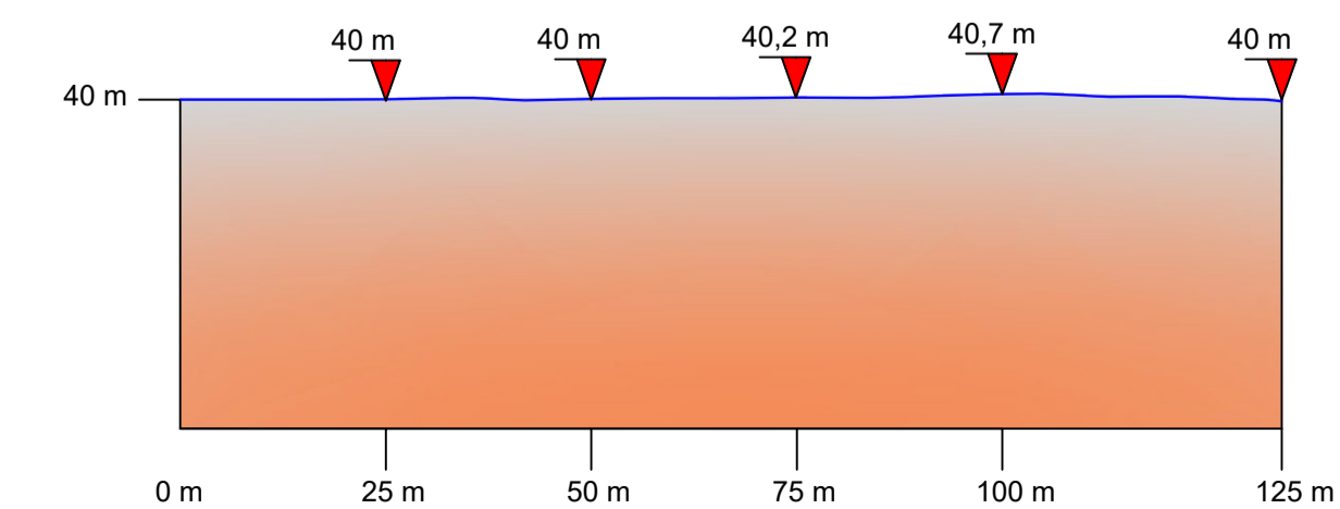
RILIEVO PLANOALTIMETRICO - TRATTO B-B'
