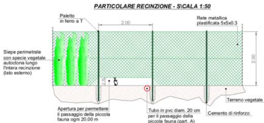
Tavola n. 4: particolare recinzione
