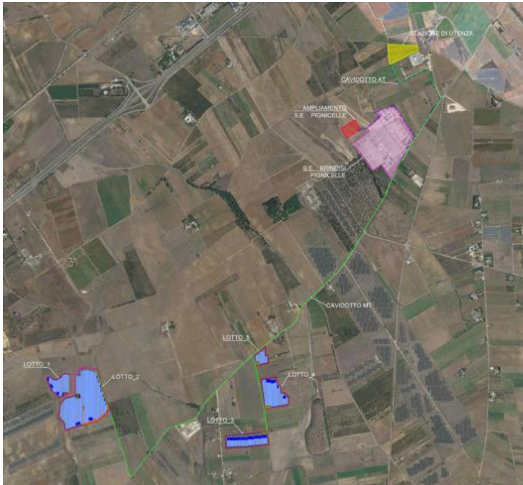
Tavola n. 5: ubicazione area impianto e sottostazione di AT esistente.
