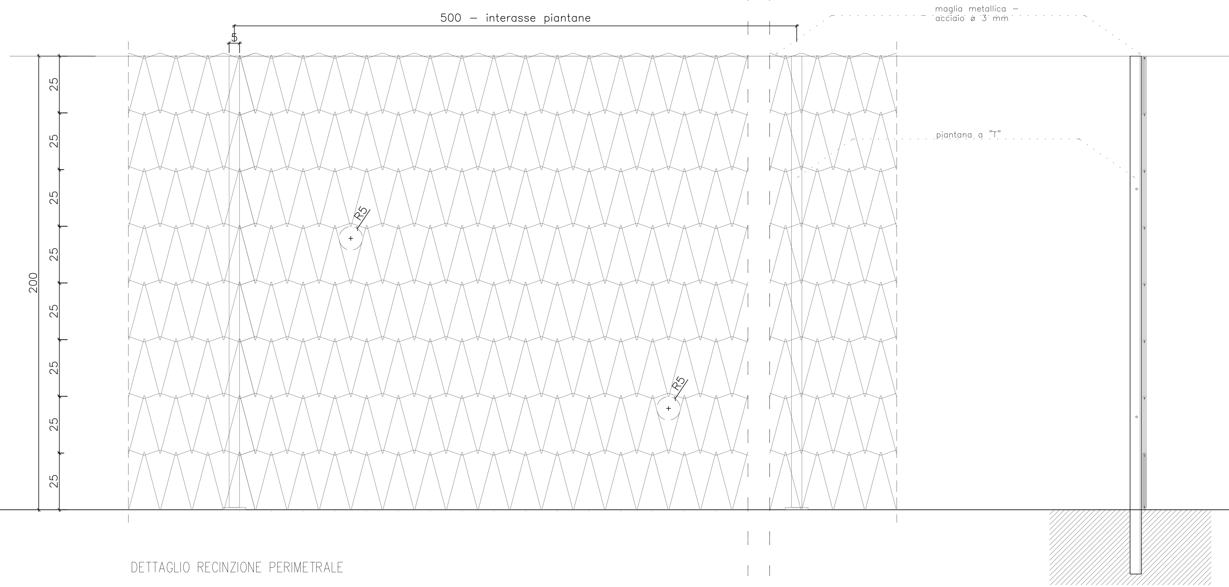
Prospetto Esterno - Rete Recinzione
