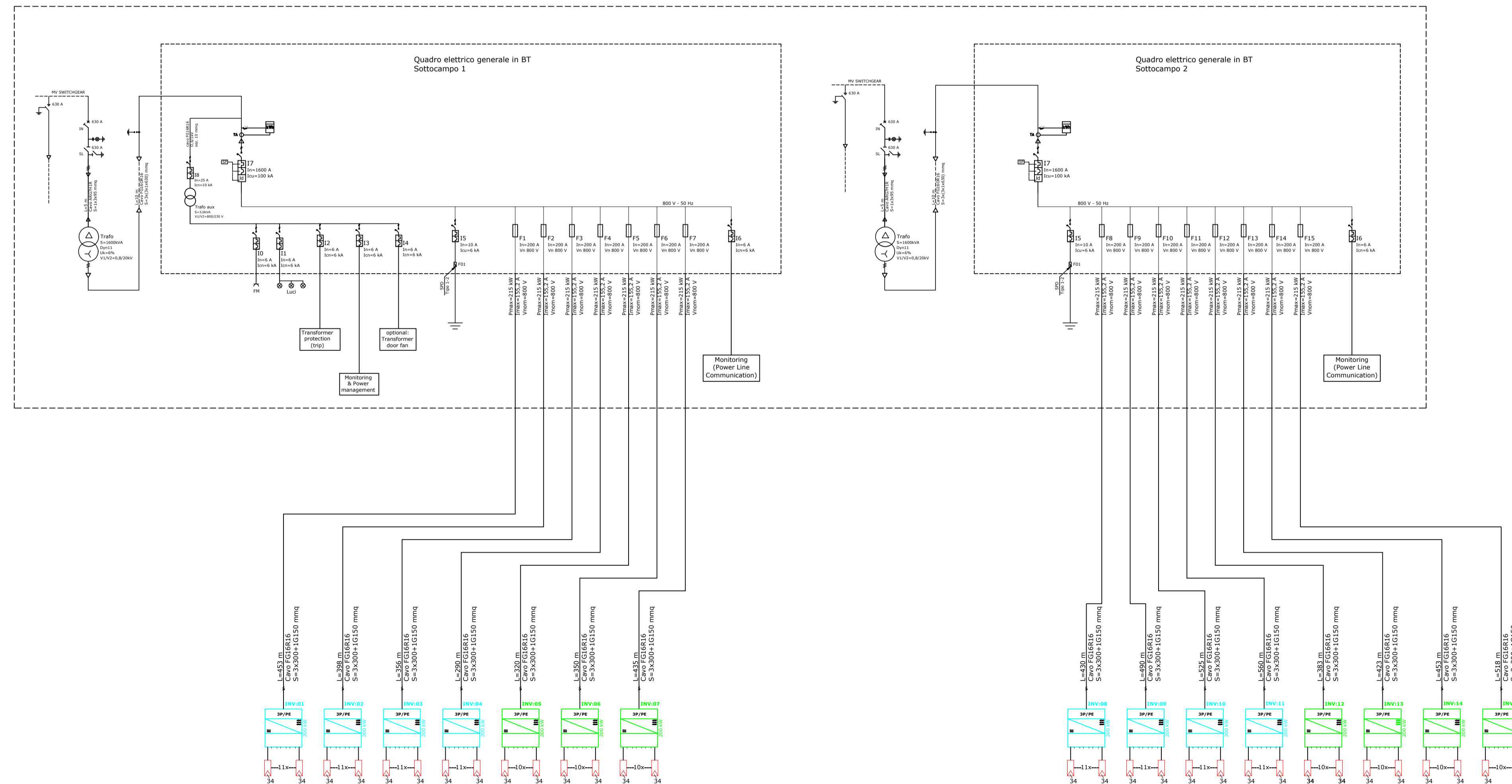
SCHEMA UNIFILARE DI COLLEGAMENTO INVERTER/QUADRO BT IN CABINA DI TRASFORMAZIONE CT1-B - IMPIANTO 1
