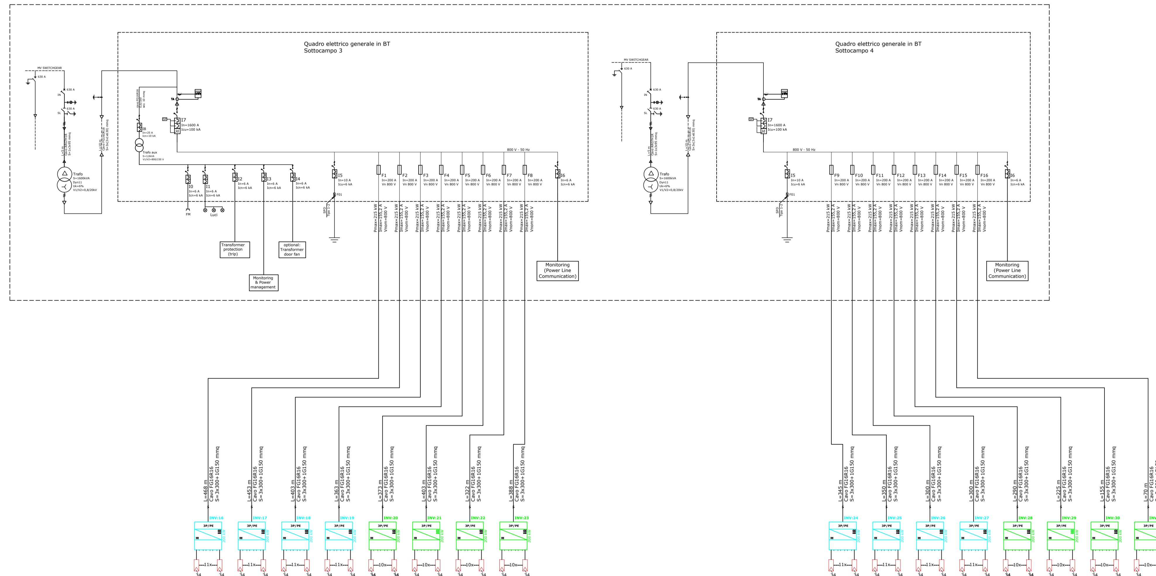
SCHEMA UNIFILARE DI COLLEGAMENTO INVERTER/QUADRO BT IN CABINA DI TRASFORMAZIONE CT1-A - IMPIANTO 1
