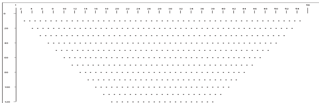
Figura 1 - Tomografia elettrica - Schema misure
