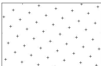
Stazioni gravimetriche
