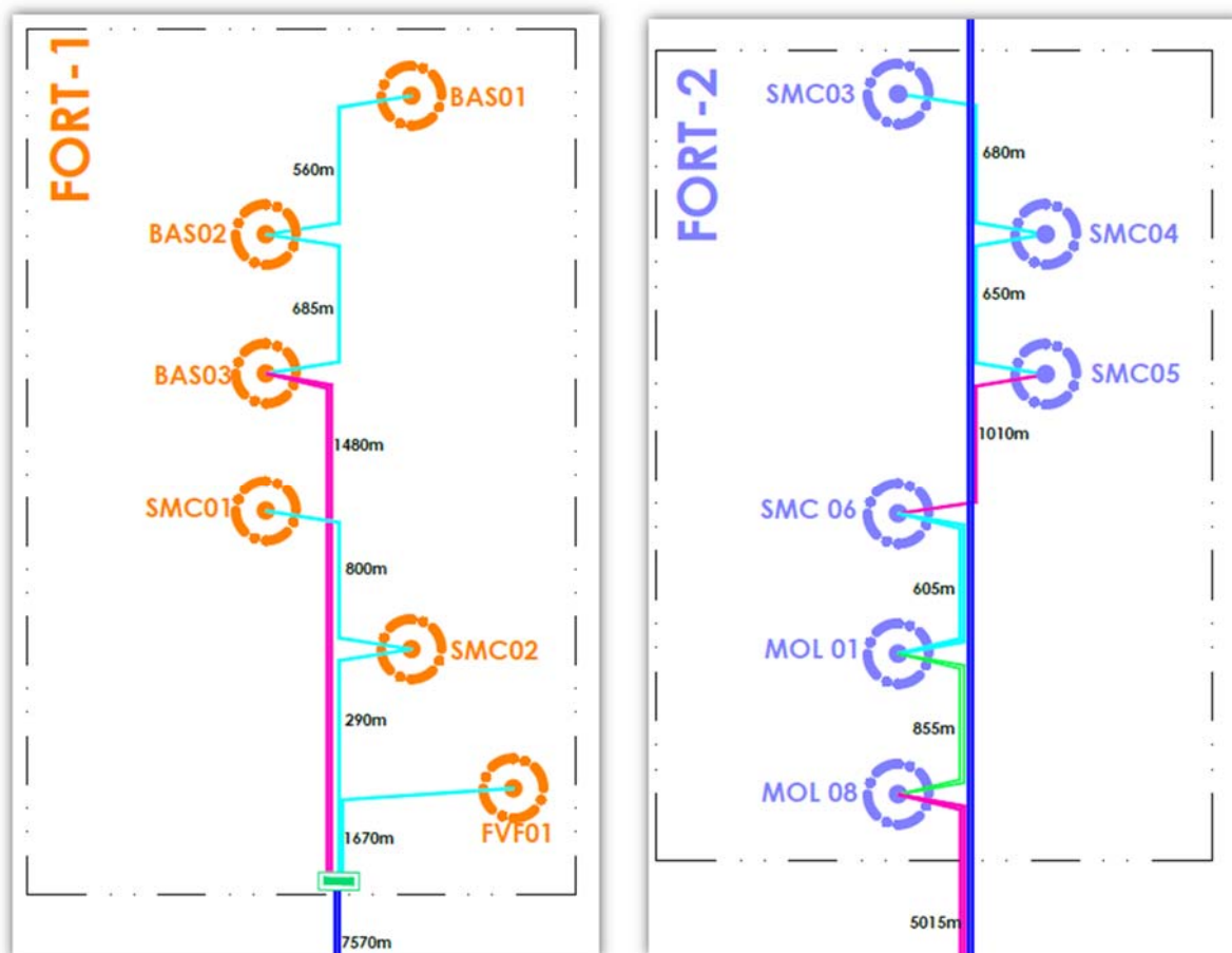
Fig. 5. Grafo a deformata delle linee MT di interconnessione degli aerogeneratori e della connessione alla RTN
