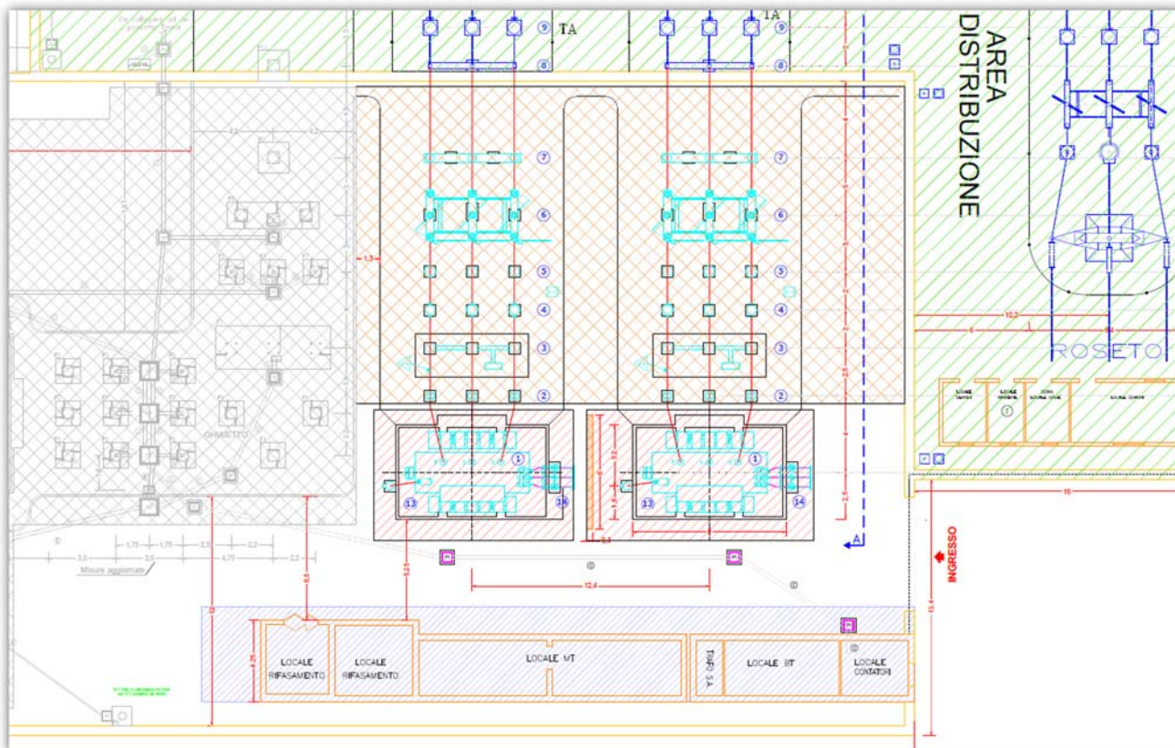
Fig. 14. Pianta elettromeccanica di dettaglio della SSE Produttore. Con campitura rossa si è indicata le vasche trafo ed i TRAFO oggetto di dismissione e sostituzione; con campitura arancio i due montanti esistenti oggetto di dismissione e rifacimento; in basso, i locali tecnici esistenti che saranno demoliti e sostituiti da 2 nuovi manufatti di tipo ad elementi prefabbricati.
