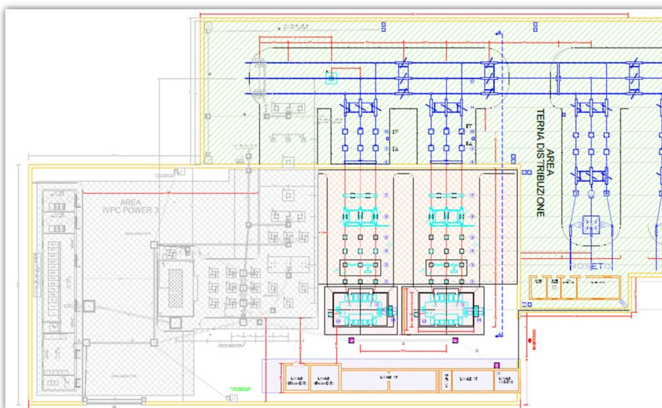
Fig. 13. Pianta elettromeccanica dell'insieme SSE Produttore-SE TERNA. Con campitura tratteggiata verde si è evidenziata la SE TERNA; con campitura grigia si sono indicate aree della SSE non oggetto di intervento. Con campitura rossa si è indicata l'area oggetto di interventi di dismissione e sostituzione; in basso, i locali tecnici esistenti che saranno demoliti e sostituiti da 2 nuovi manufatti di tipo ad elementi prefabbricati.
