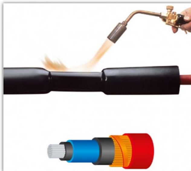
Fig. 7. – Schema di esecuzione di un giunto MT
