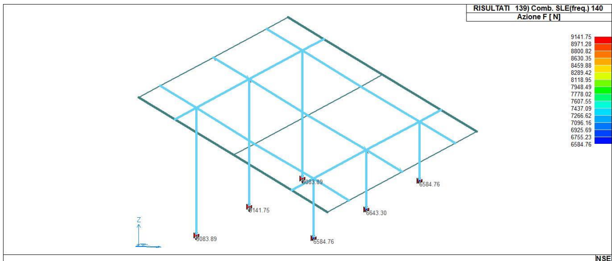
42_RIS_REAZIONI_139_Comb. SLE(freq.) 140
