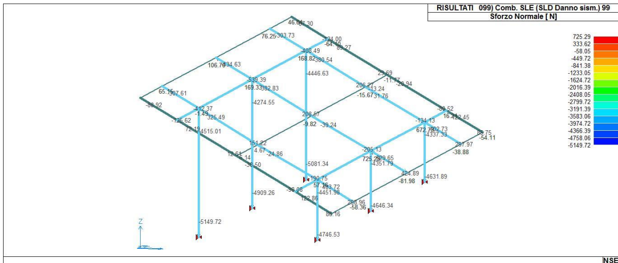
43_RIS_N_099_Comb. SLE (SLD Danno sism.) 99
