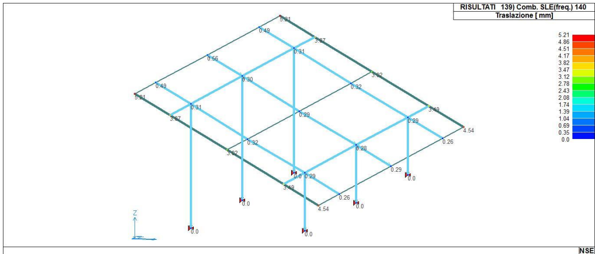
41_RIS_SPOSTAMENTI_139_Comb. SLE(freq.) 140
