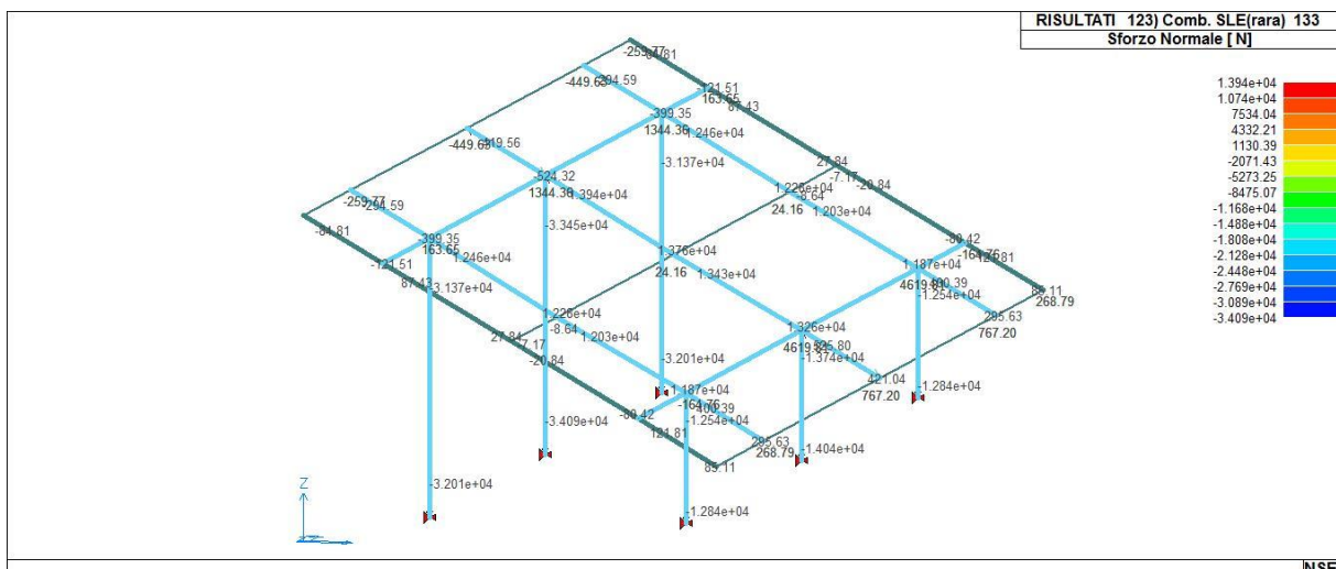
43_RIS_N_123_Comb. SLE(rara) 133
