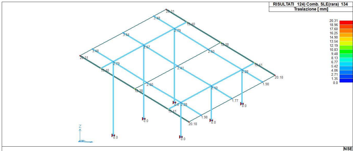
41_RIS_SPOSTAMENTI_124_Comb. SLE(rara) 134
