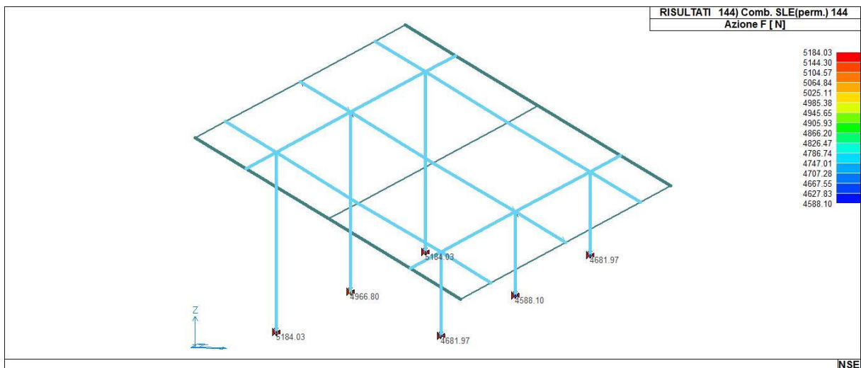
42_RIS_REAZIONI_144_Comb. SLE(perm.) 144
