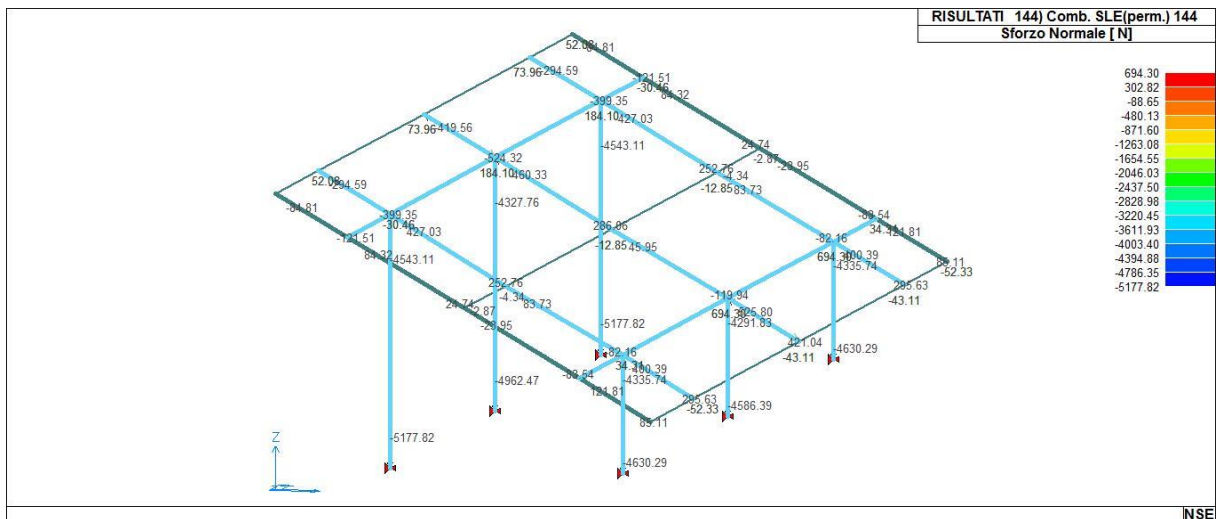
43_RIS_N_144_Comb. SLE(perm.) 144
