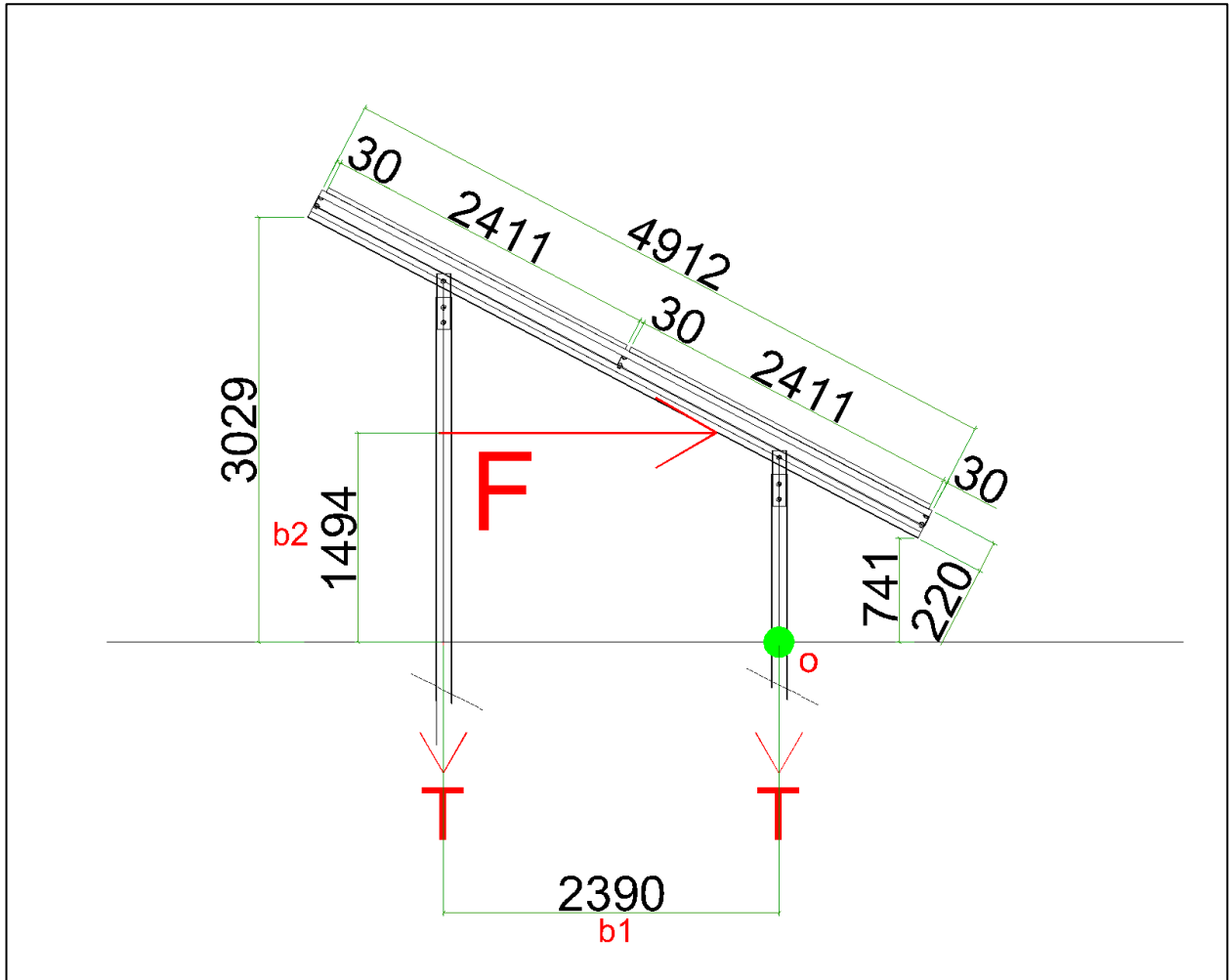
Figura: Schema di ribaltamento della struttura
