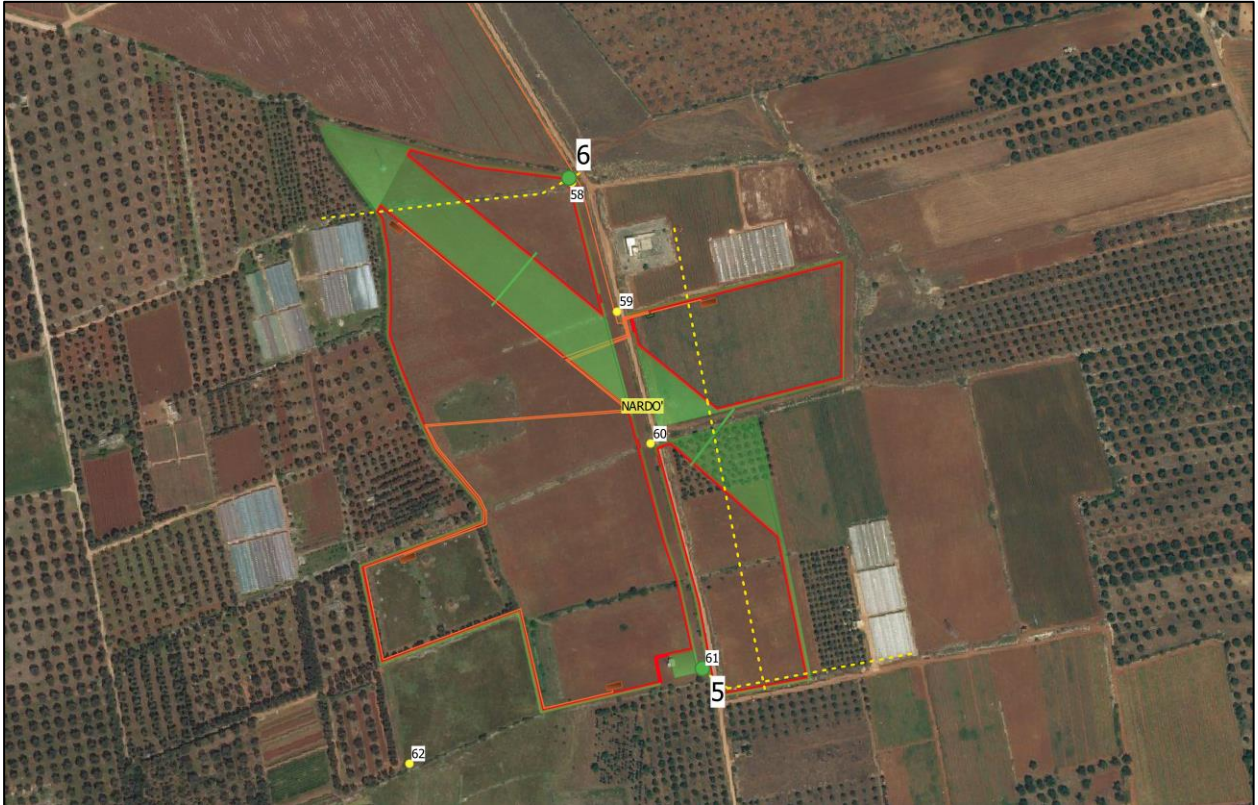
Planimetria punti di scatto demolizione linee aeree
