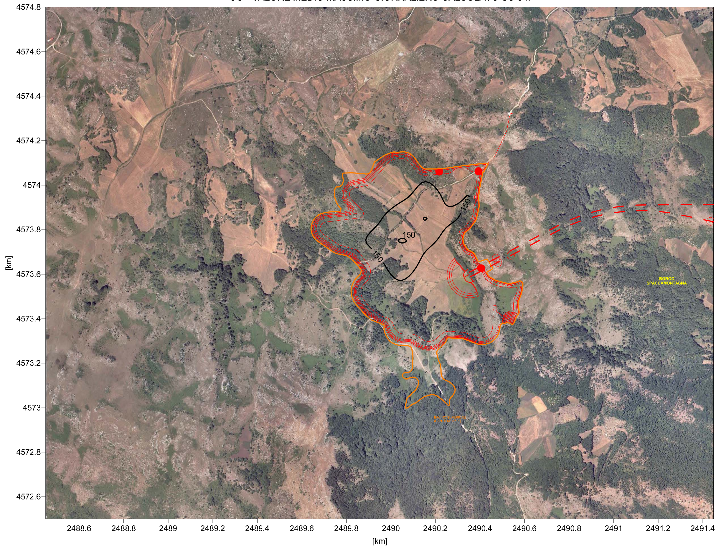
FIGURA 2.3 CANTIERE No. 1 MAPPA DELLE CONCENTRAZIONI DI INQUINANTI AL LIVELLO DEL SUOLO CO VALORE MEDIO MASSIMO GIORNALIERO CALCOLATO SU 8 h
