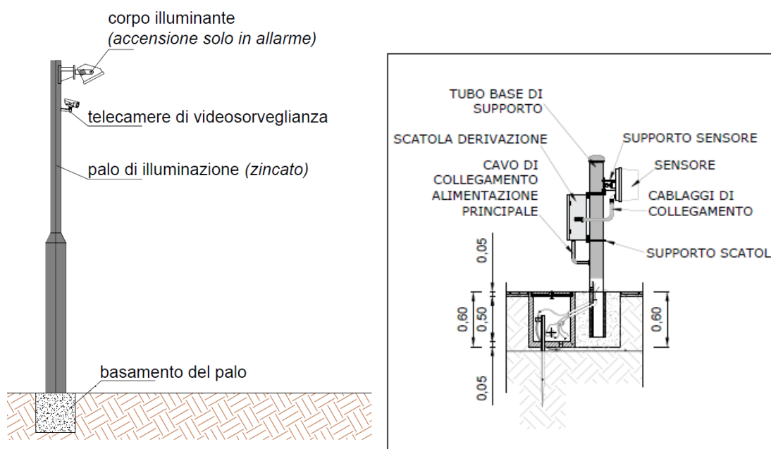
Fig. 24 – Sistema antintrusione
