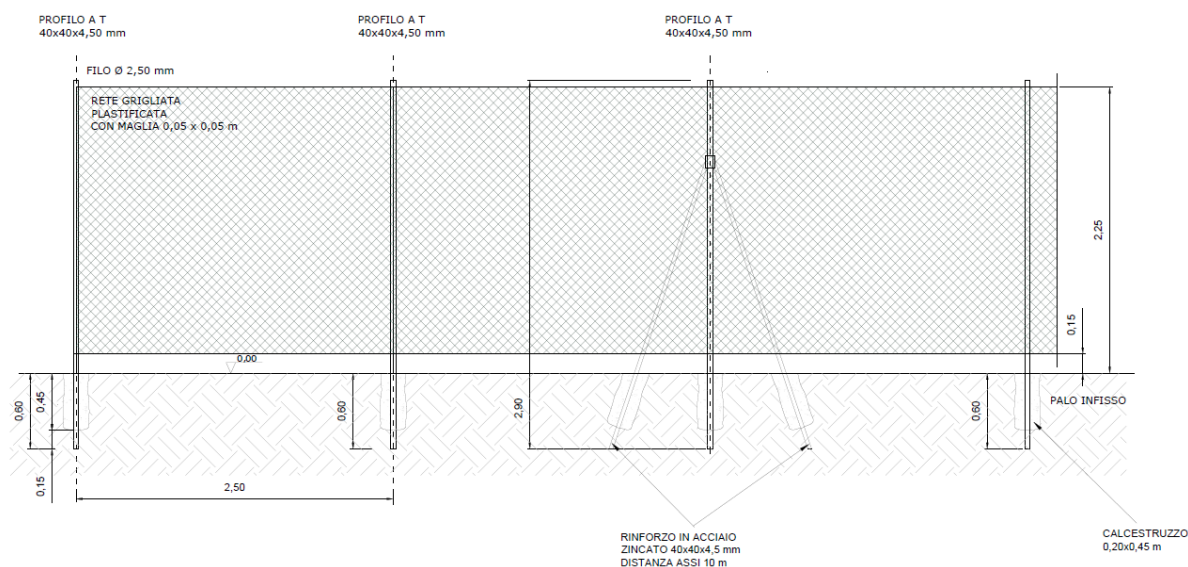
Fig. 18 – Recinzione perimetrale
