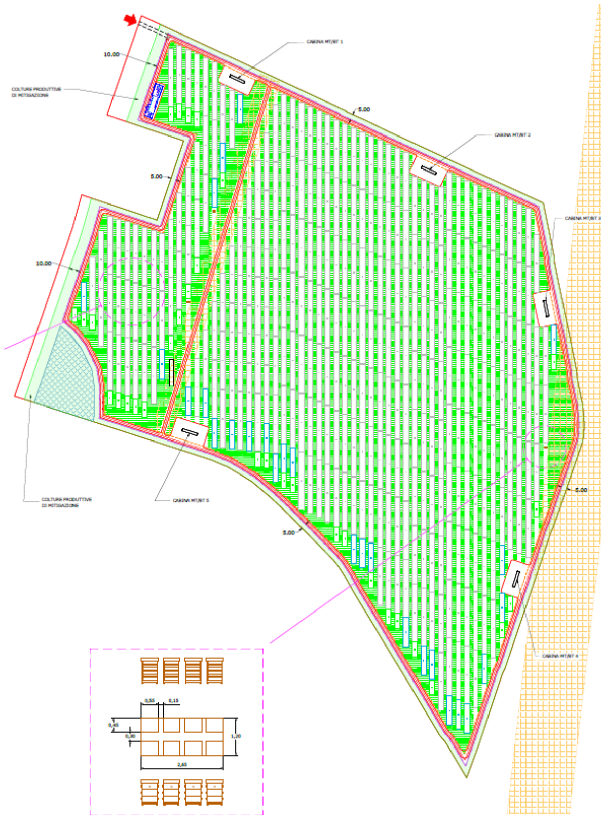
Fig. 4 – Area di impianto agrosolare
