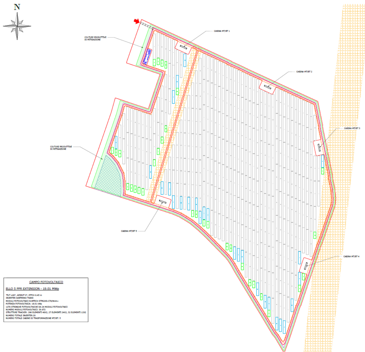
Fig. 7 - Layout di impianto
