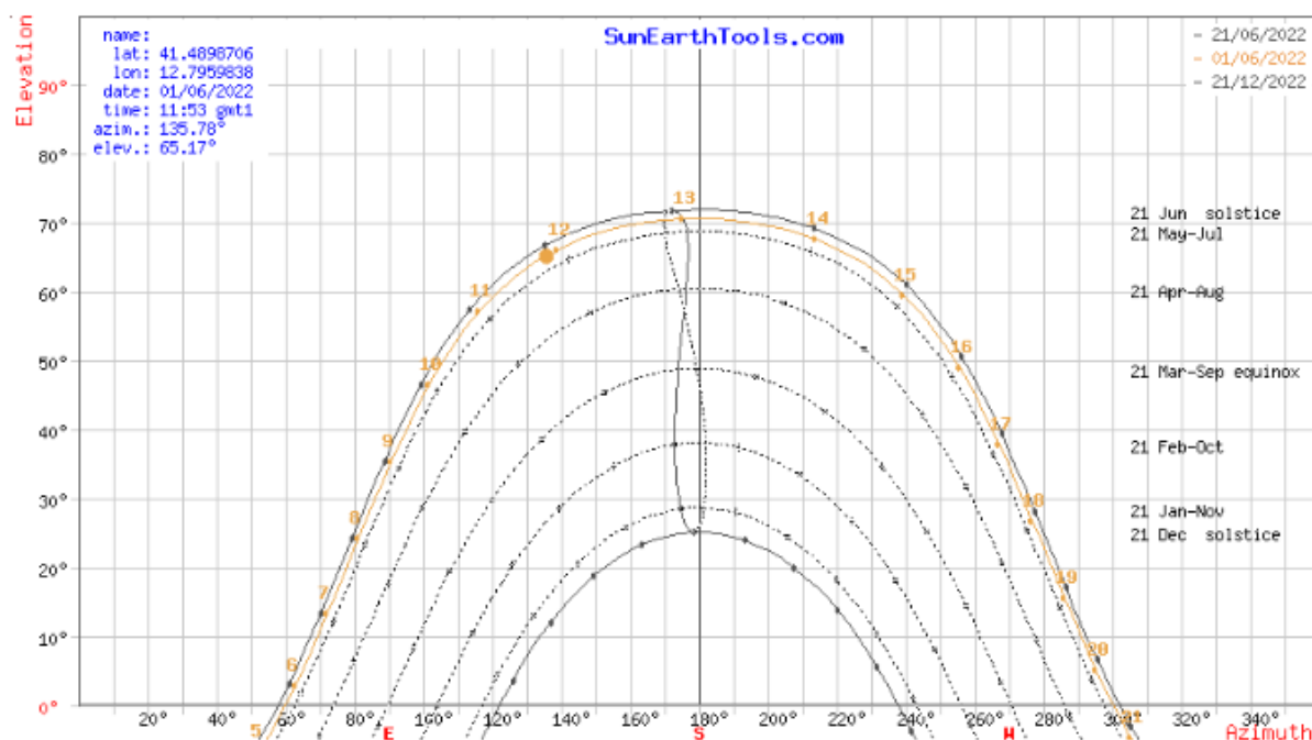
Fig. 28 - Diagramma Solare Polare (riferito al sito di Castelverde)
