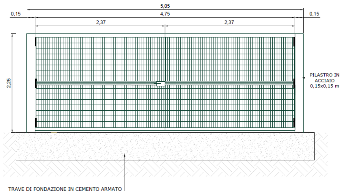
Fig. 19 – Cancello a doppia anta
