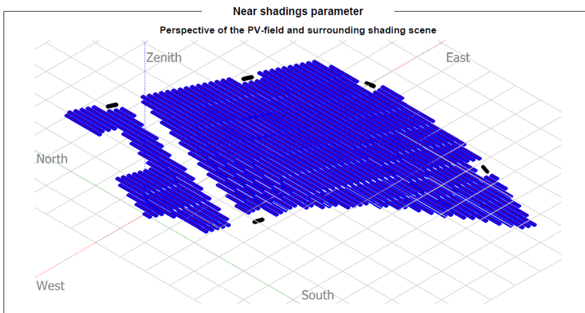
Fig. 29 – Diagramma delle ombre
