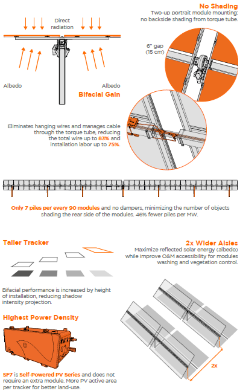
Fig. 12 - Dimensioni, specifiche tecniche e prestazionali Inseguitori solari (Tracker)
