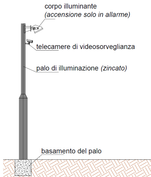
Fig. 25 – Sistema di illuminazione
