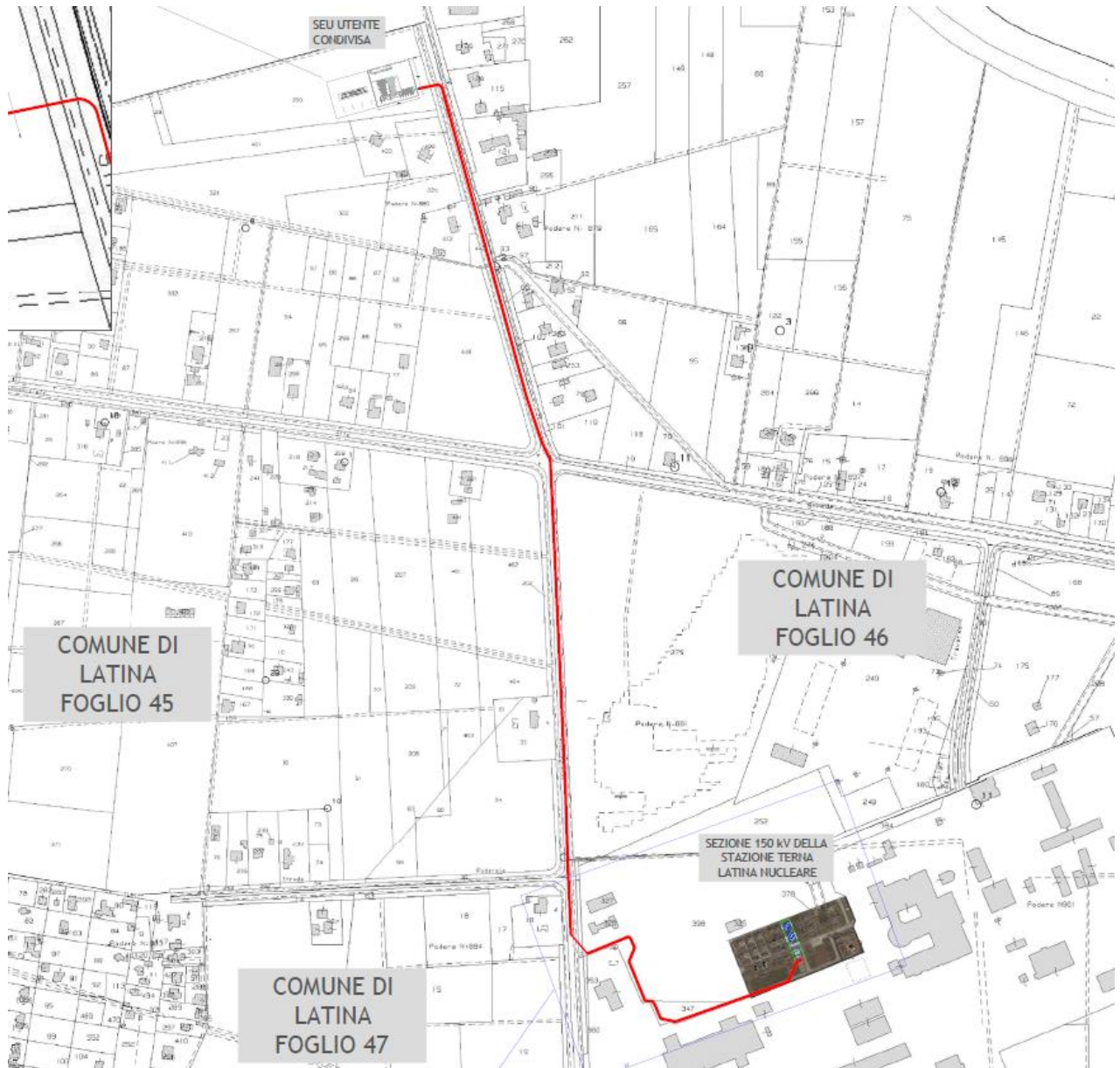
Fig. 10 – Collegamento in cavo AT tra SEU e SE Latina Nucleare
