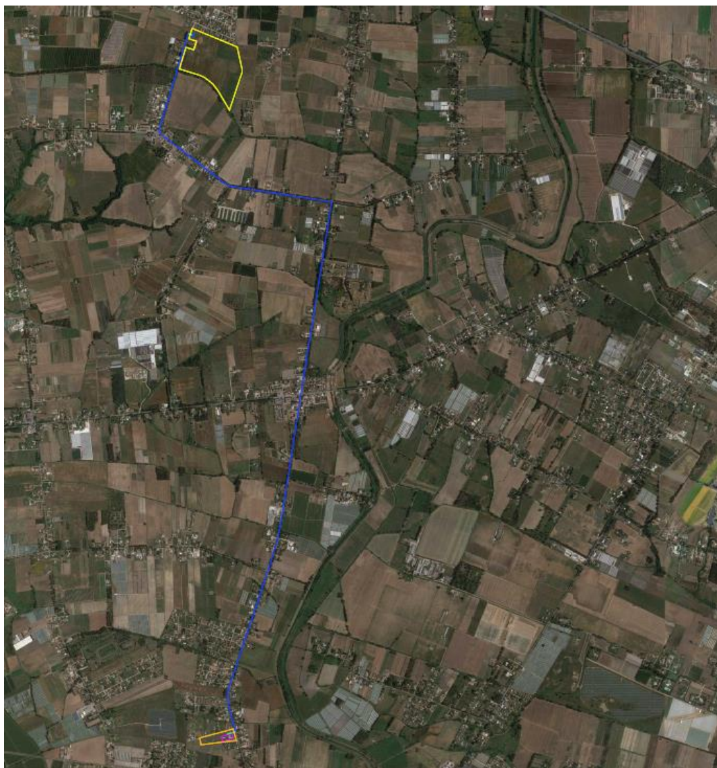
Fig. 8 – Collegamento in cavo MT su ortofoto
