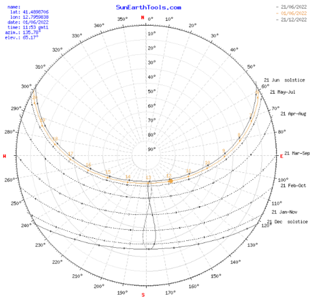
Fig. 27 - Diagramma Solare Polare (riferito al sito di Castelverde)
