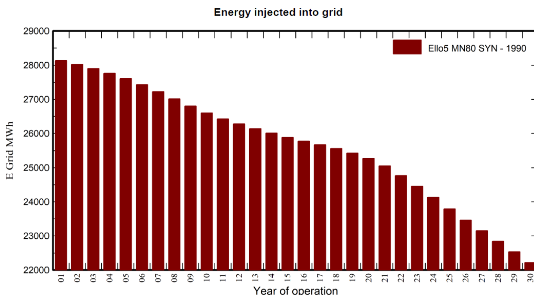
Fig. 31 – Producibilità dell’impianto con degrado moduli (30 anni)
