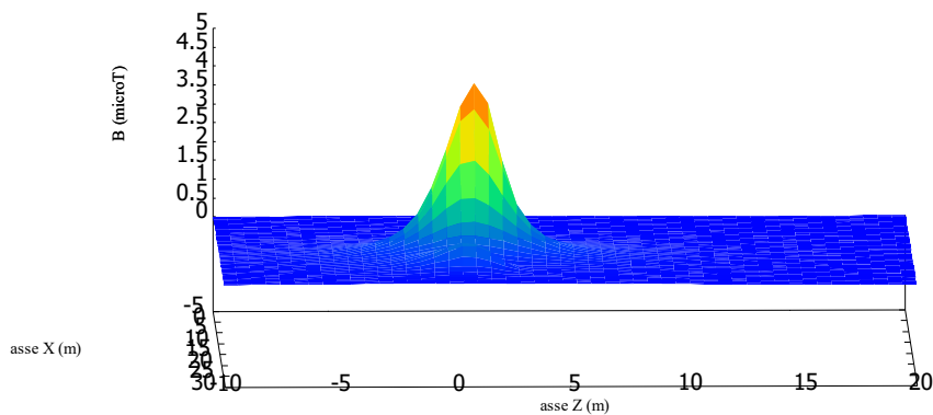
Cabina - calcolo su piano xz - quote Y=-1 m
