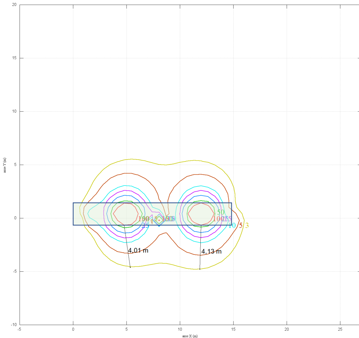
Cabina - calcolo su piano xy - quote Z=1,27 m
