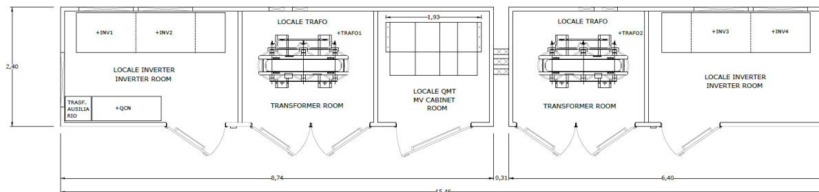
Fig.4 - Ingombri cabine di trasformazione MT/BT
