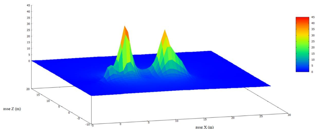
Cabina - calcolo su piano xz - quote Y=-1 m
