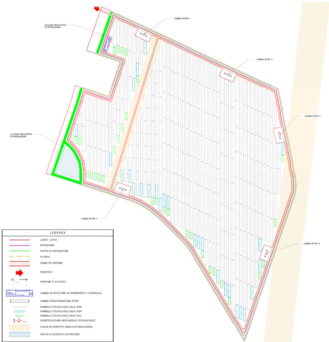
Immagine 2: Planimetria dell'impianto
