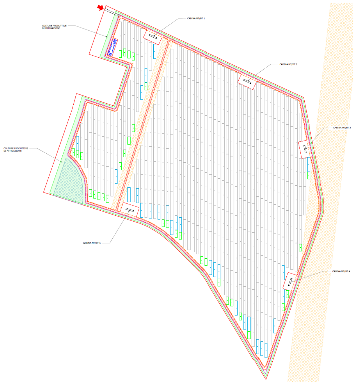
Fig. 4 - Layout di impianto
