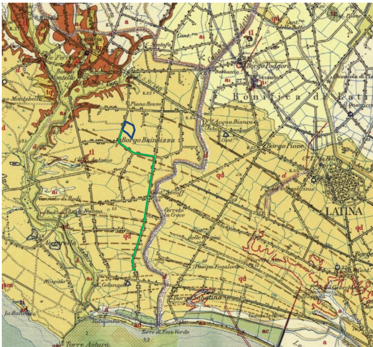
FIG. 5 - CARTA GEOLOGICA
