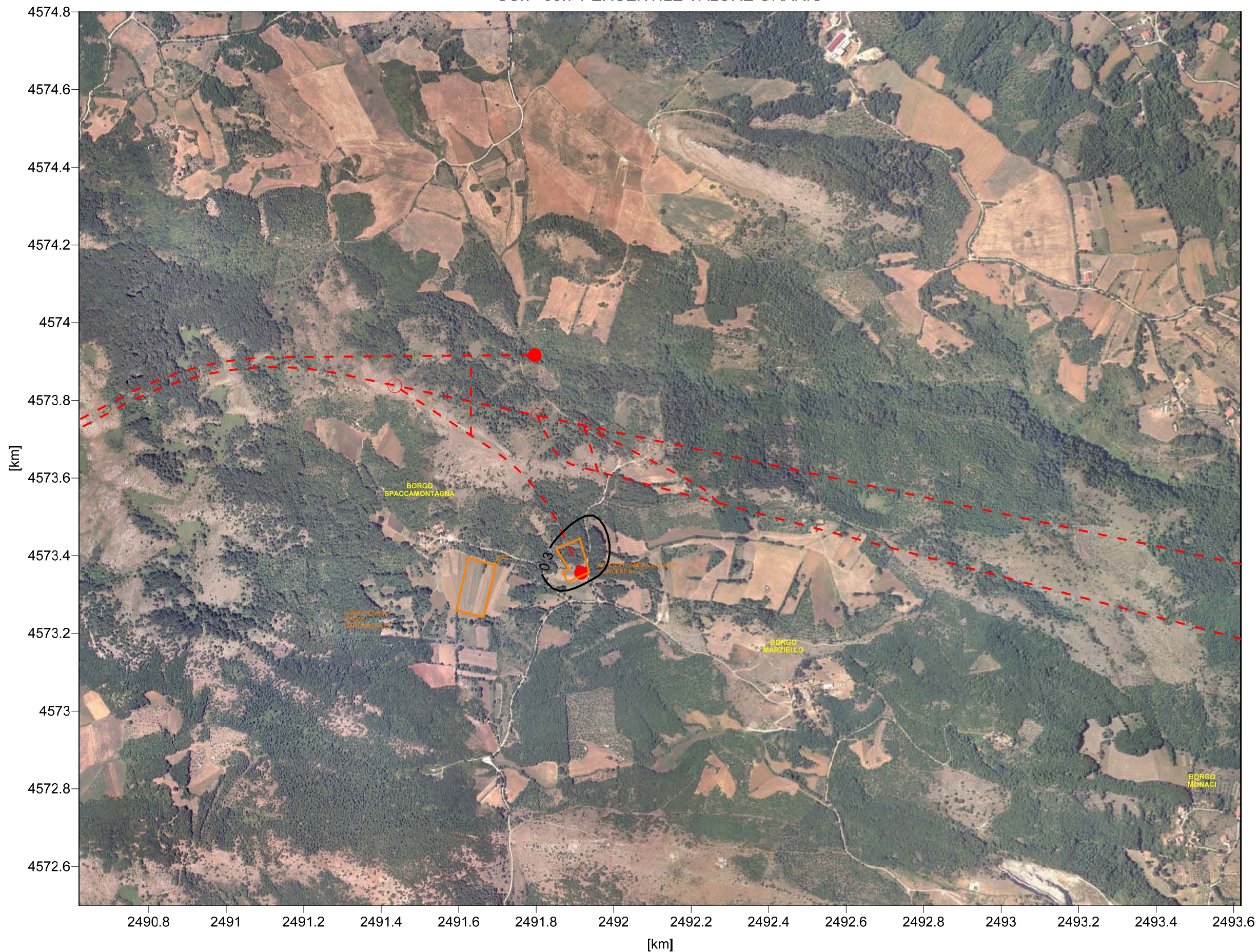
FIGURA 2.13 CANTIERE No. 2 MAPPA DELLE CONCENTRAZIONI DI INQUINANTI AL LIVELLO DEL SUOLO SOx 99.7 PERCENTILE VALORE ORARIO
