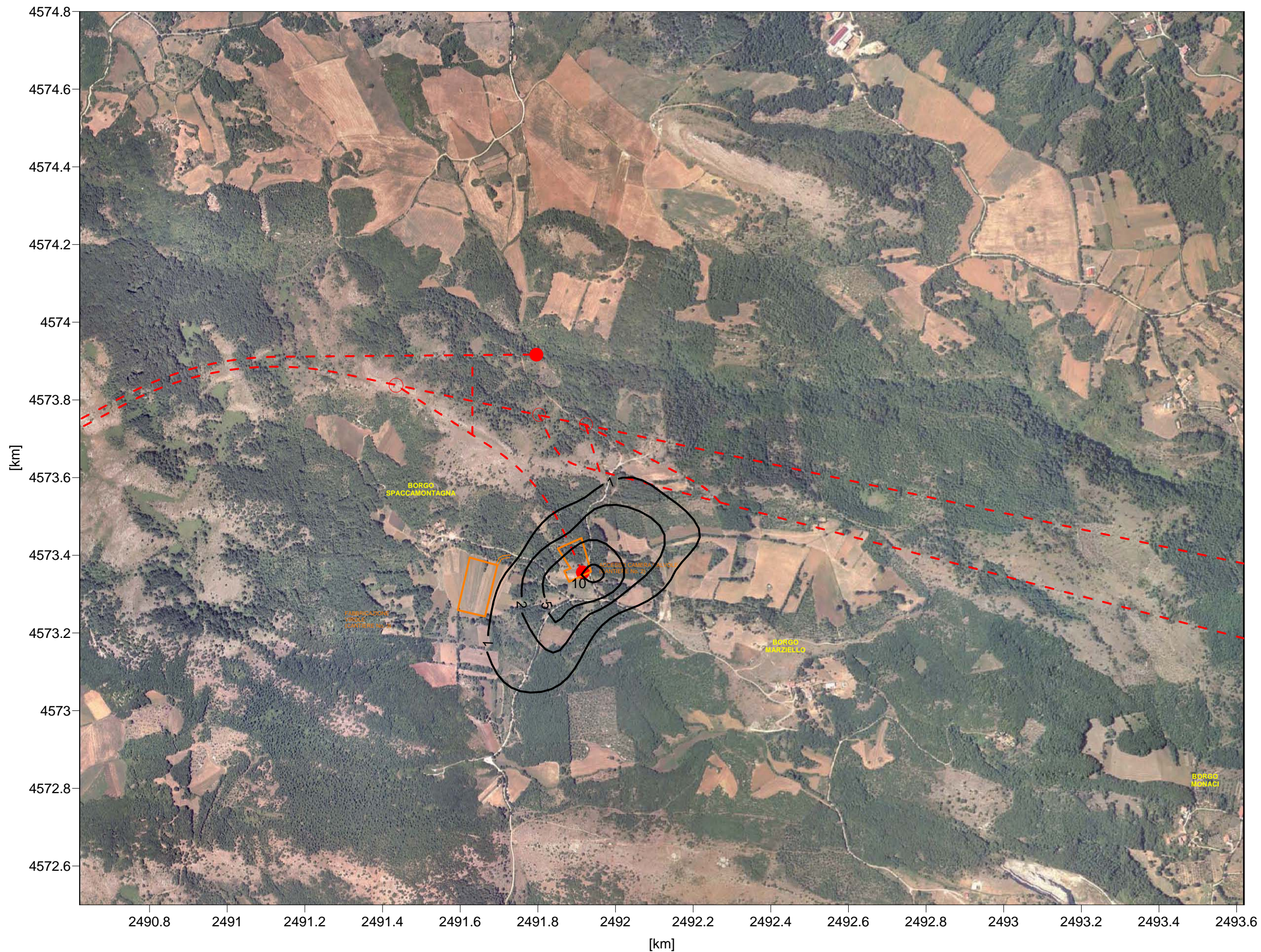
FIGURA 2.15 CANTIERE No. 2 MAPPA DELLE CONCENTRAZIONI DI INQUINANTI AL LIVELLO DEL SUOLO PM10 VALORE MEDIO ANNUO
