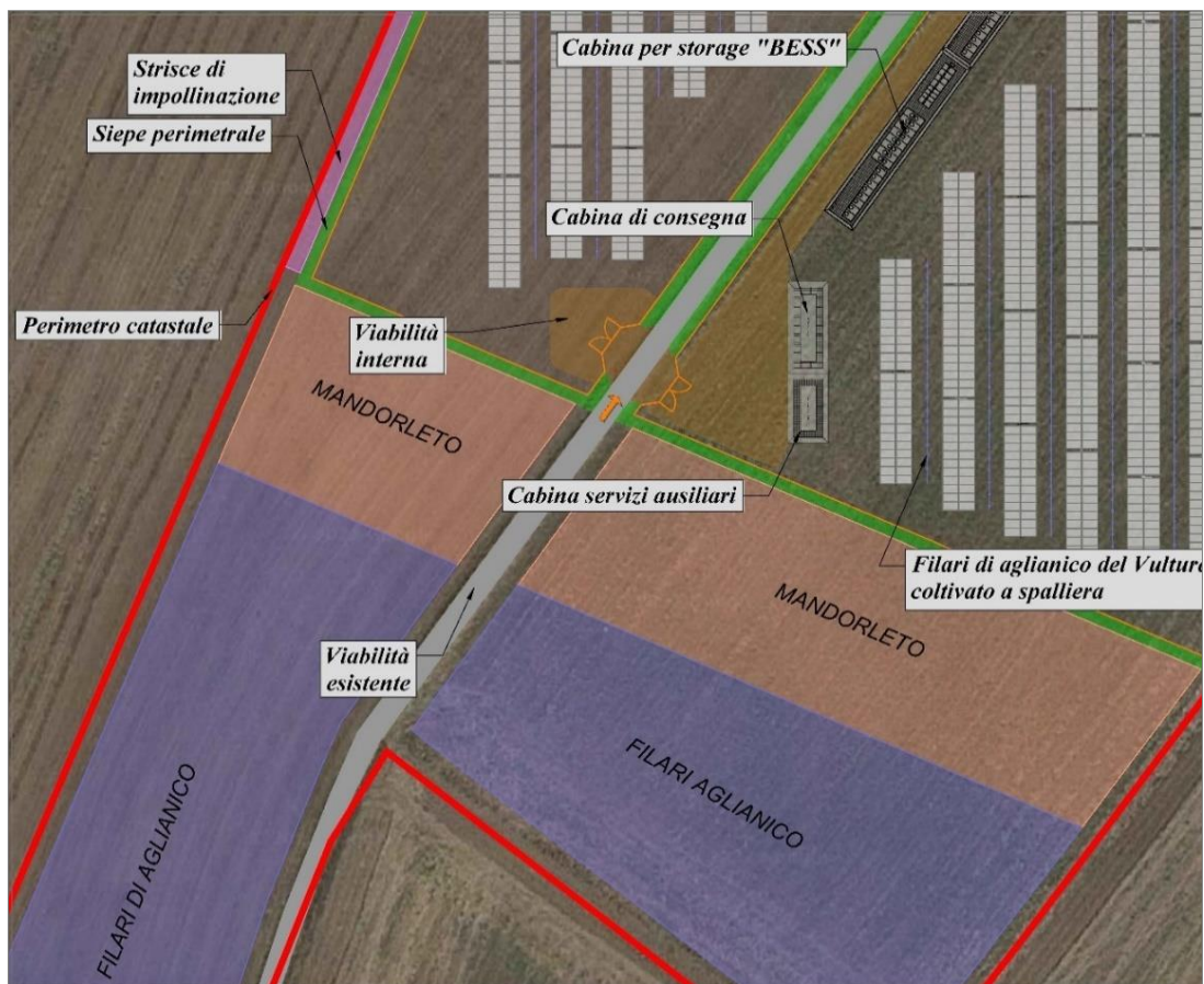
Stralcio planimetrico con indicazione delle mitigazioni previste
