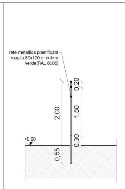
SEZIONE TIPO
