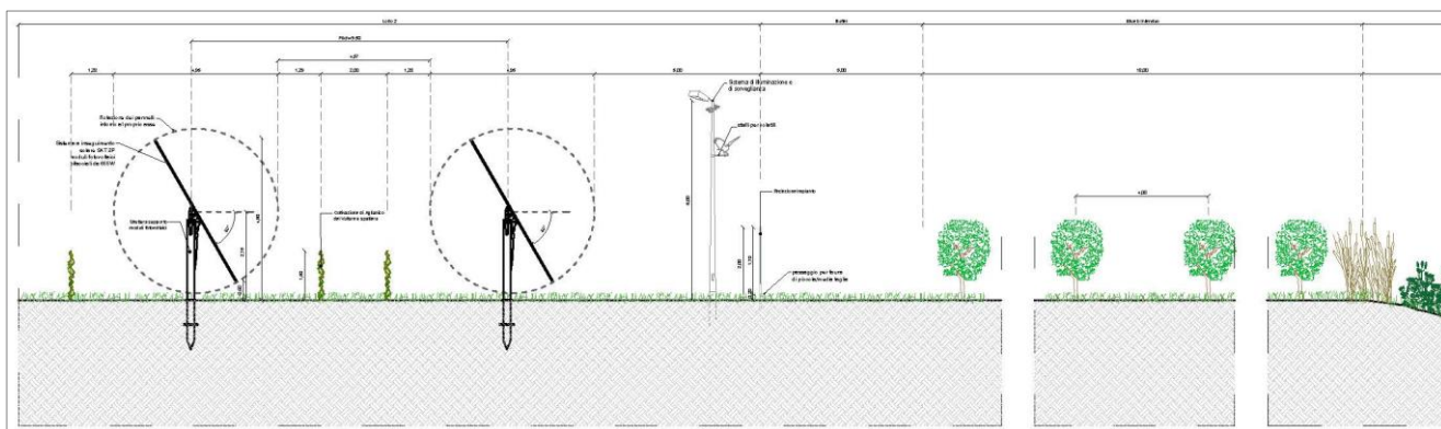
Sezione progettuale con indicazione delle mitigazioni previste
