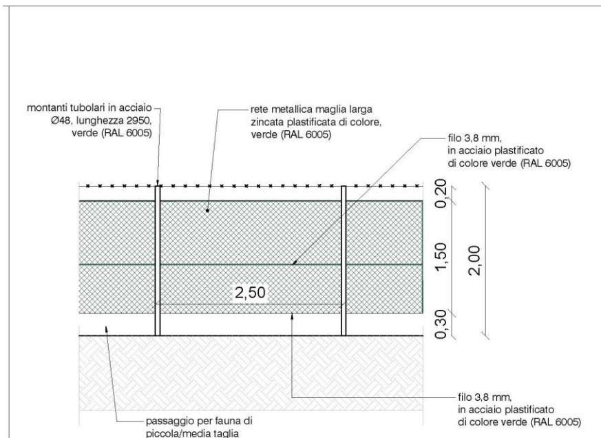
PROSPETTO TIPO
