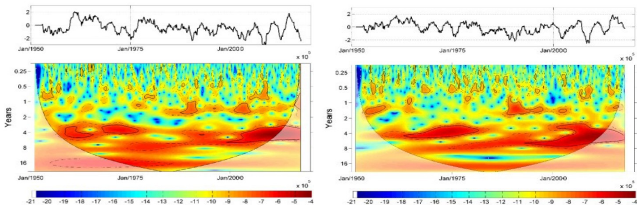
Figura 9 - Wavelet Analysis applicata alle serie temporali di SPI24 (1951-2017) per il versante tirrenico. Il grafico nel pannello superiore mostra l'andamento dell'SPI24 analizzato (a destra per il versante tirrenico a sinistra per quello adriatico)
