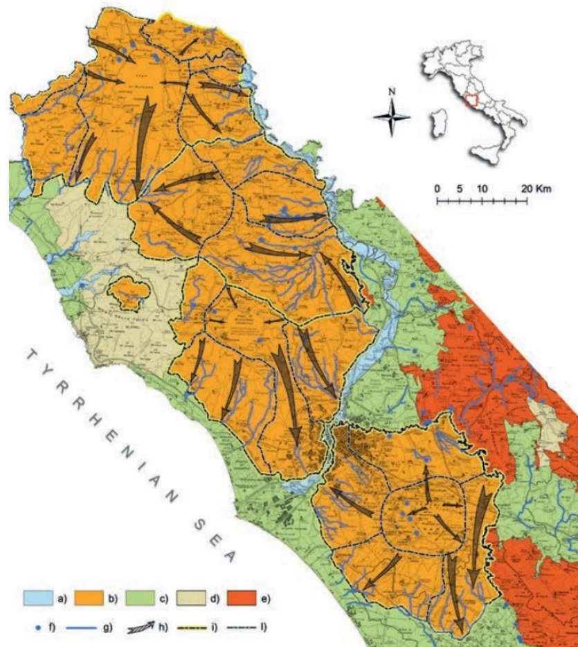
Figura 13 - Schema delle unità idrogeologiche del dominio vulcanico laziale – (Capelli et al., 2012b modificato) Legenda: a) Unità alluvionali; b) Unità vulcaniche; c) Unità detritico – alluvionali; d) Unità flyschoidi; e) Unità carbonatiche; f) sorgenti puntuali con portata media superiore a 50 L/s; g) sorgenti lineari con portata media superiore a 50 L/s; h) principali direttrici di flusso idrico sotterraneo; i) limiti delle unità idrogeologiche vulcaniche; l) limite dei bacini idrogeologici vulcanici. (Tratto da L'idrogeologia regionale nella pianificazione e gestione della risorsa idrica sotterranea. Il dominio vulcanico laziale (Italia centrale) - Acque Sotterranee - Italian Journal of Groundwater (2013))
