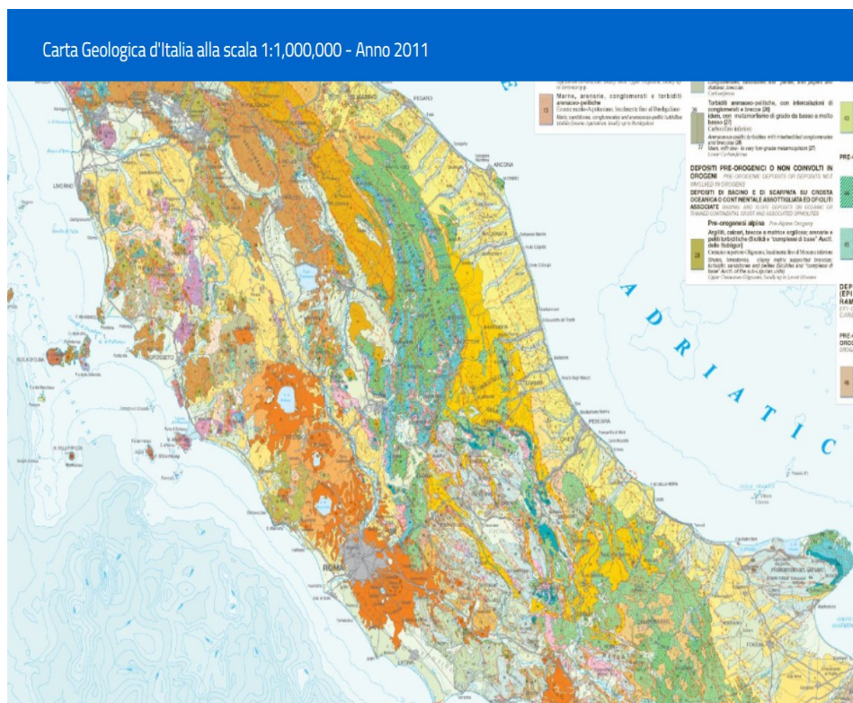
Figura 10 - Carta geologica d'Italia in scala 1:1.000.000 (Compagnoni et al. 2011)
