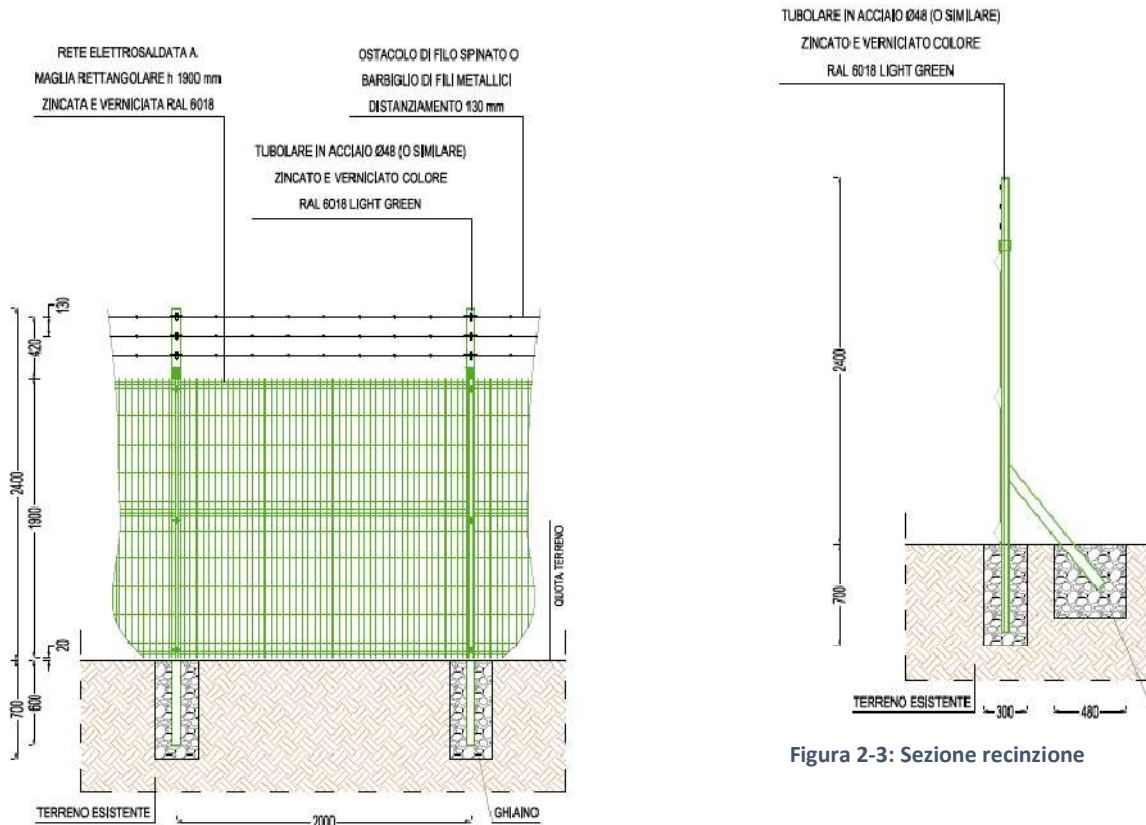
Figura 2-2: Prospetto recinzione
