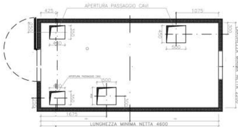
Figura 2-17: Pianta chioschi
