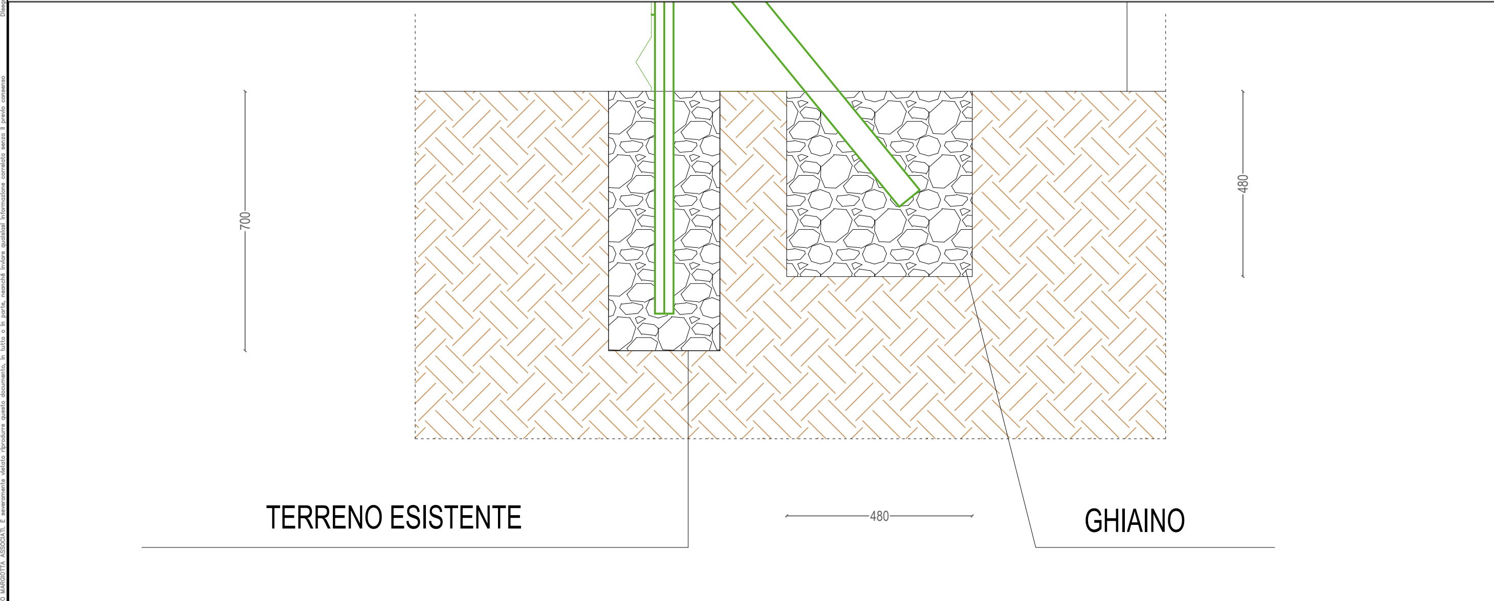
DETTAGLIO E_Ancoraggio recinzione scala 1:50
