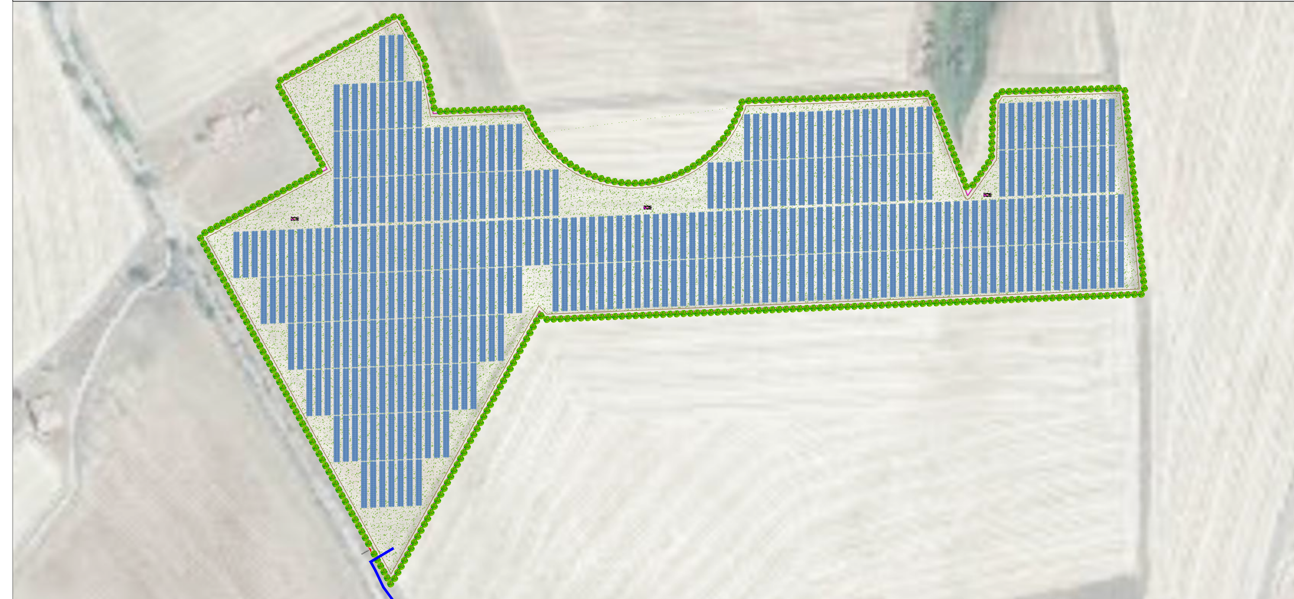
STRALCIO PLANIMETRICO CAMPO AGRIVOLTAICO scala 1:2000
