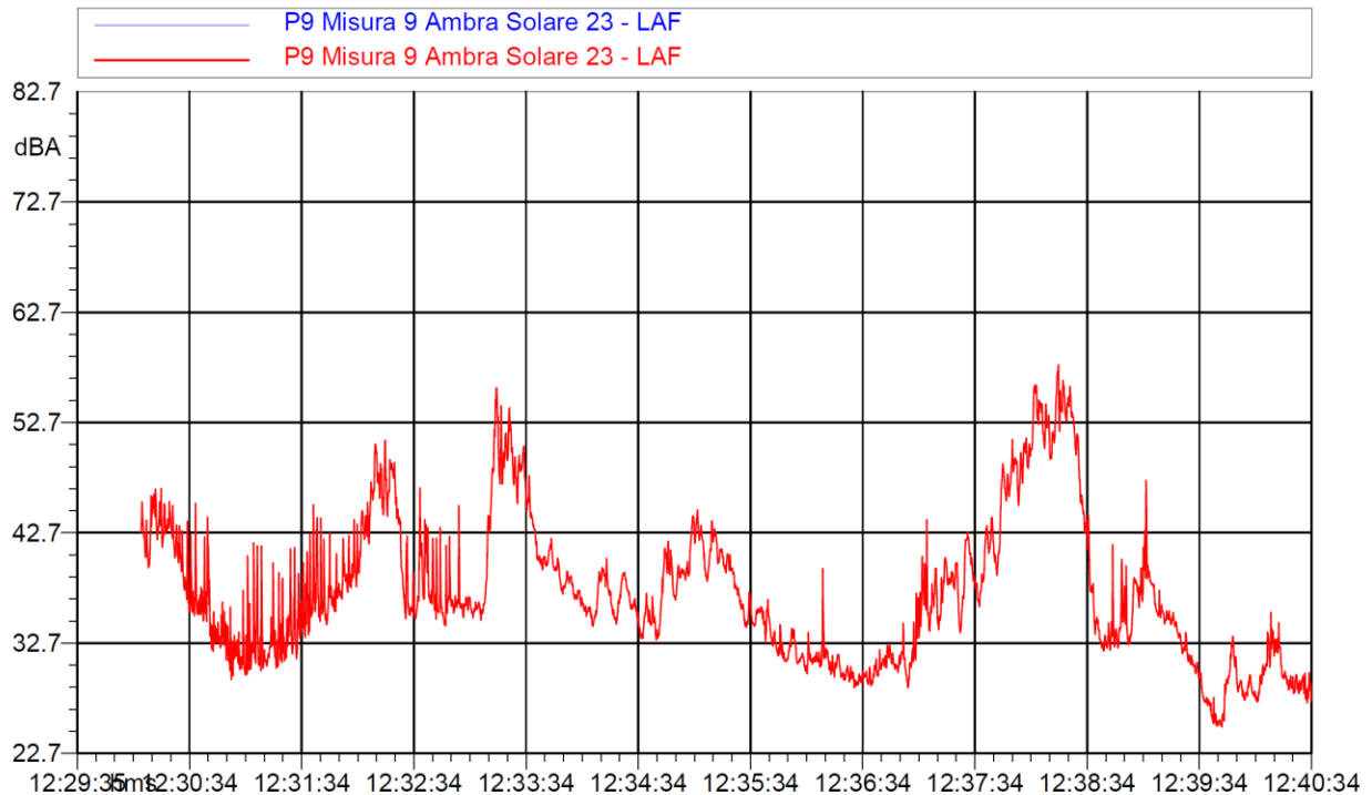
Fig. 26 - Time history e tabella dati della misura M9 nel punto P9 – Recettore 7
