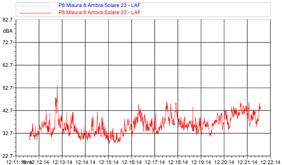
Fig. 24 - Time history e tabella dati della misura M8 nel punto P8 – Recettore 6
