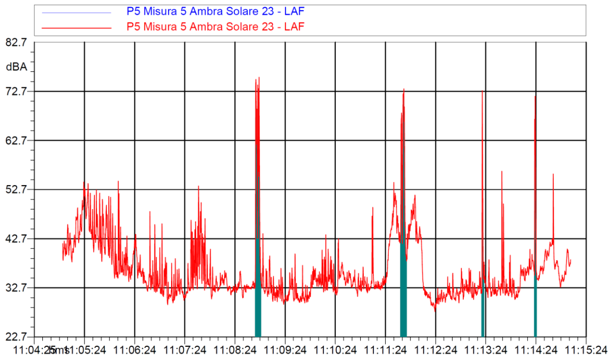
Fig. 17- Time history e tabella dati della misura M5 nel punto P5
