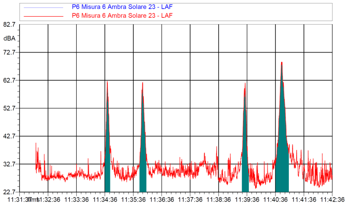
Fig. 20 - Time history e tabella dati della misura M6 nel punto P6 – Recettore 4
