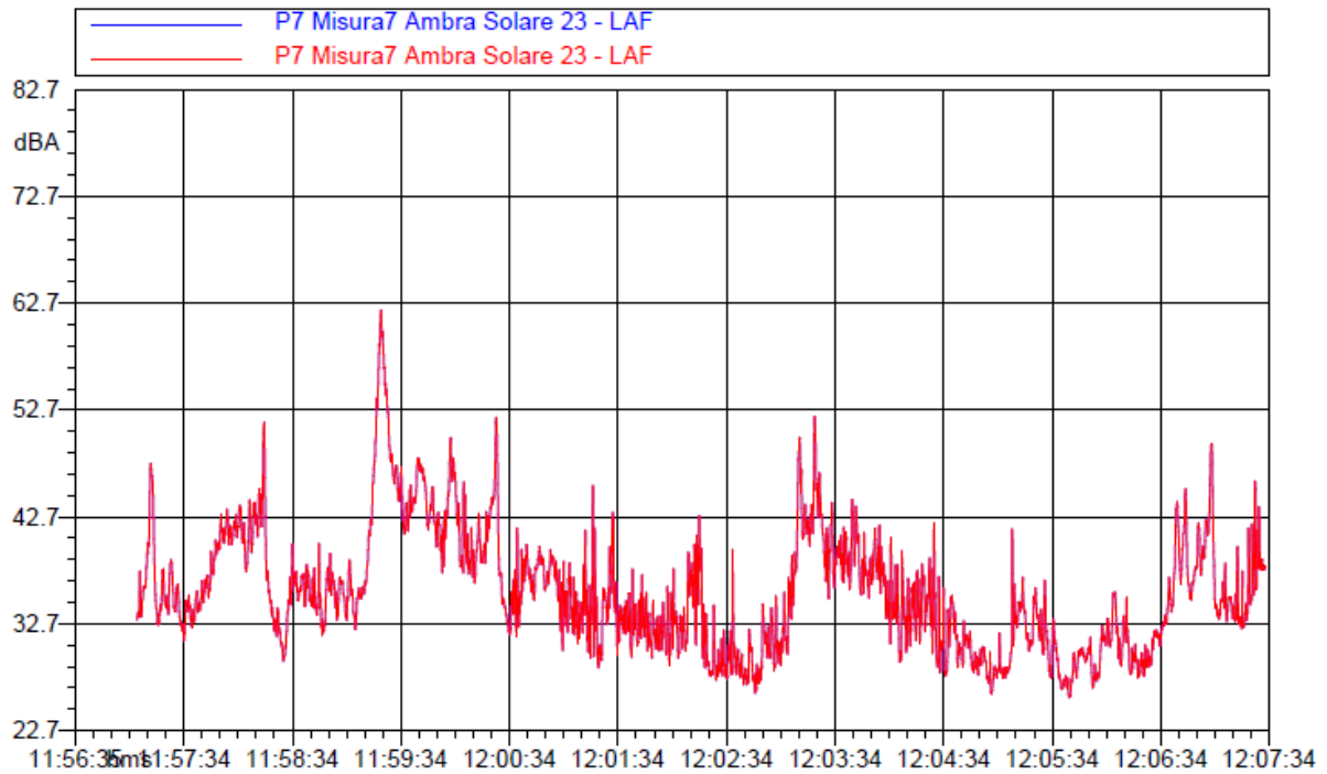
Fig. 22 - Time history e tabella dati della misura P7 – Recettore 5
