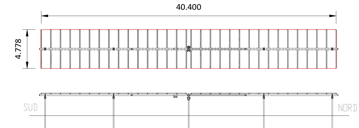
Fig. 5 – Vista laterale e vista dall'alto traker tipo
