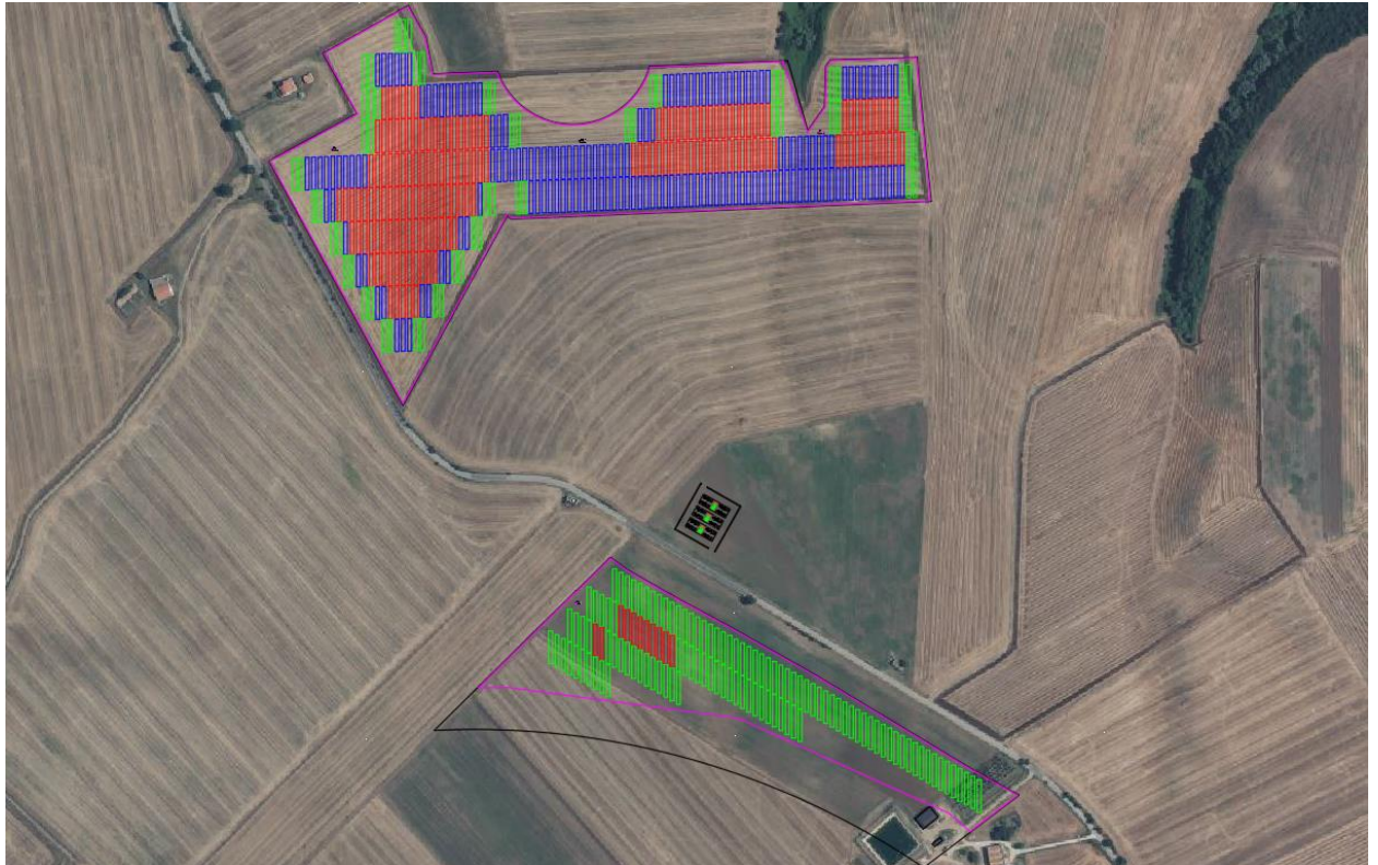
Fig. 6 – Disposizione generale impianto
