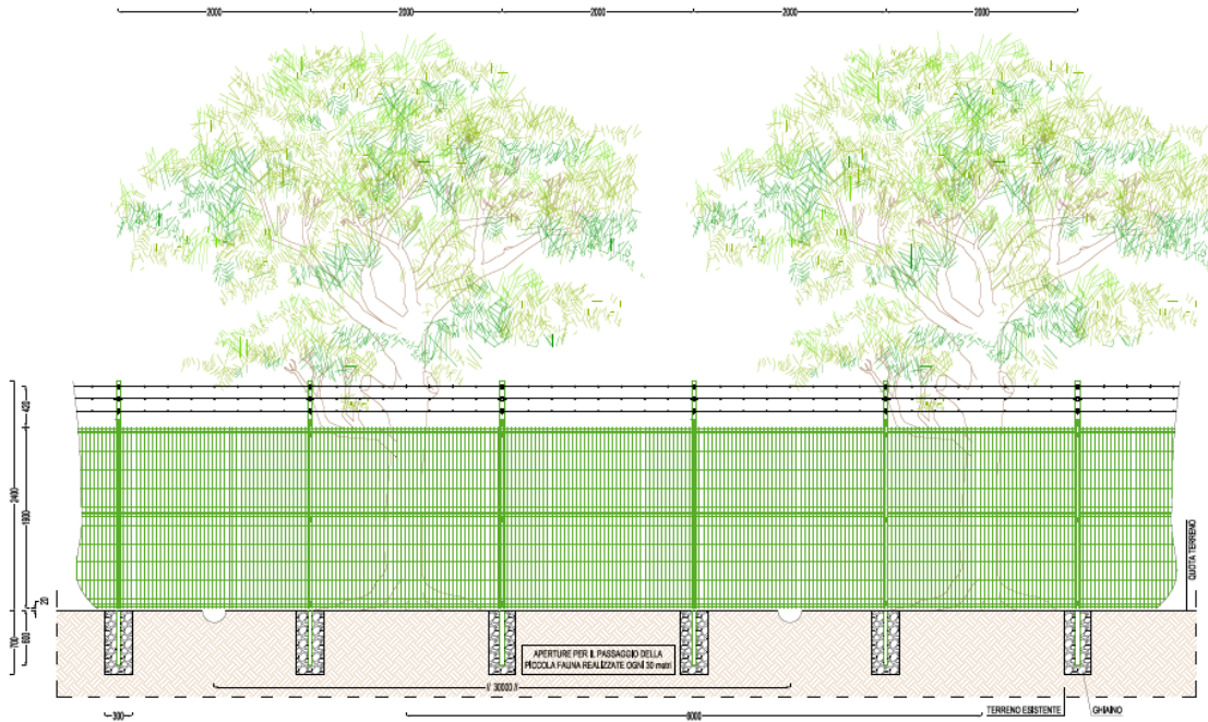
Figura 11: Prospetto recinzione con fascia di mitigazione
