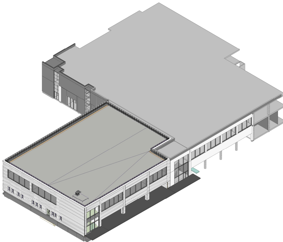
Fig. 11 Vista 3D del modello, prospetto air side/prospetto sud ovest
