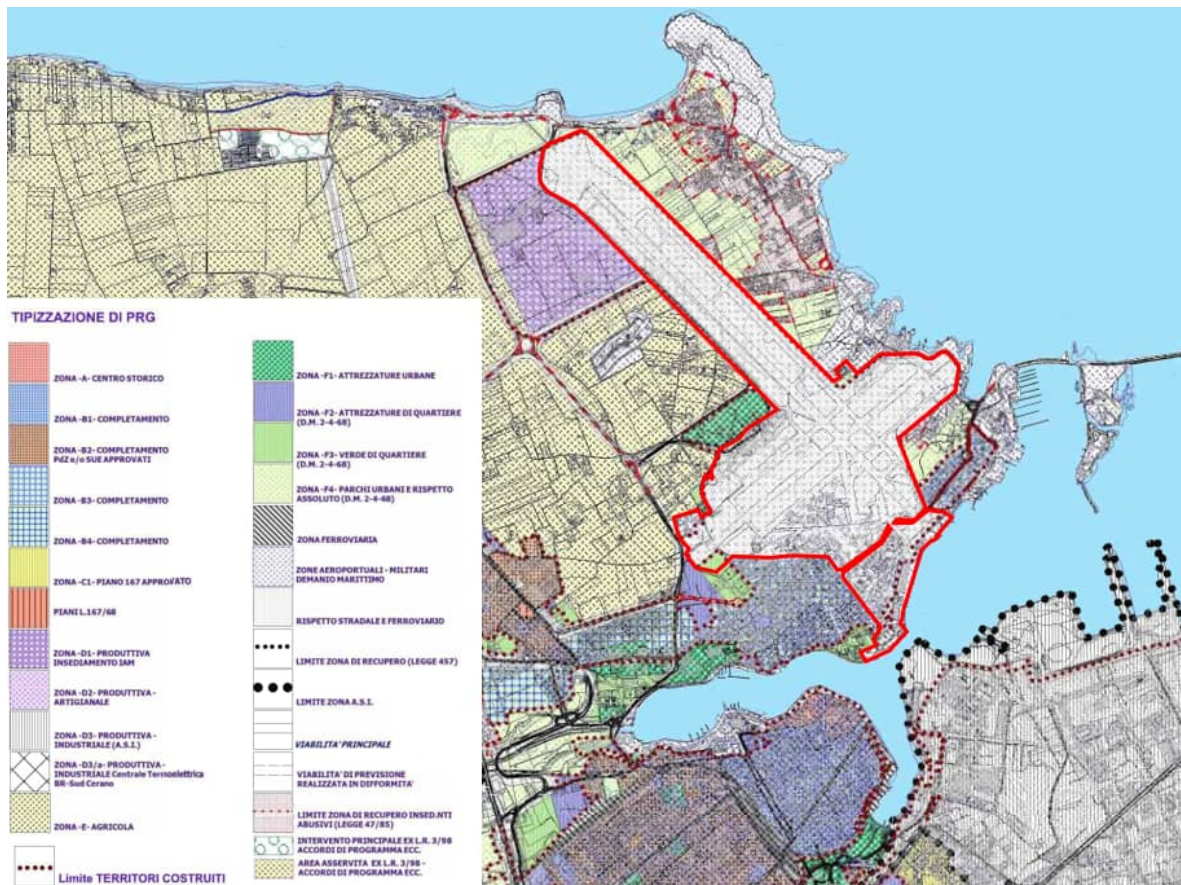
Fig. 8 Estratto della tavola n. 01A dell'adeguamento del PRG al PUTT/P, con in rosso i confini del sedime aeroportuale
