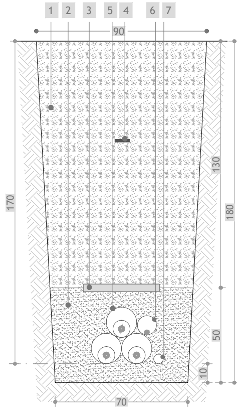
DETTAGLIO C
