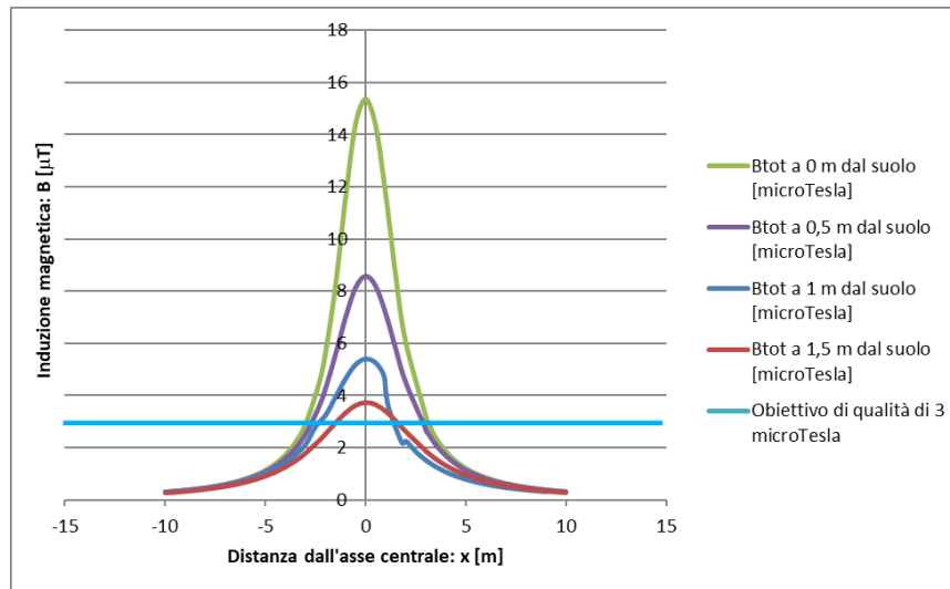
Figura 3: Andamento del campo magnetico generato dal cavidotto, composto da quattro terne da 630 mm 2 più due terne da 300 mm 2
