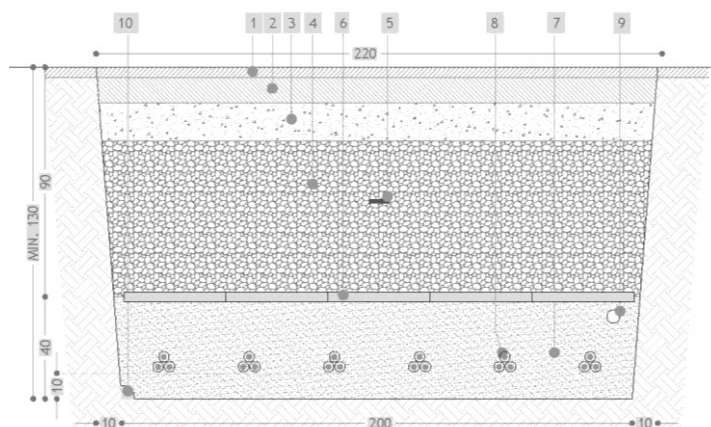
Figura 2: Sezione tipo cavidotto composta da da quattro terne da 630 mm 2 più due terne da 300 mm 2
