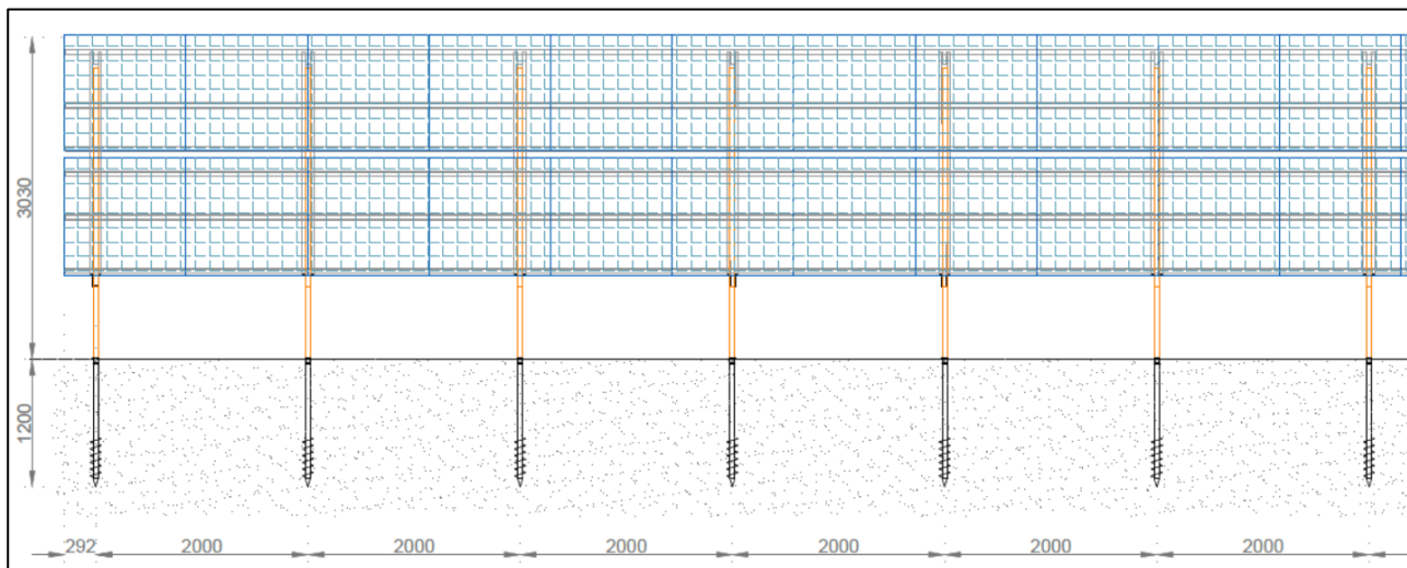
Figure 3: stralcio prospetto struttura di supporto
