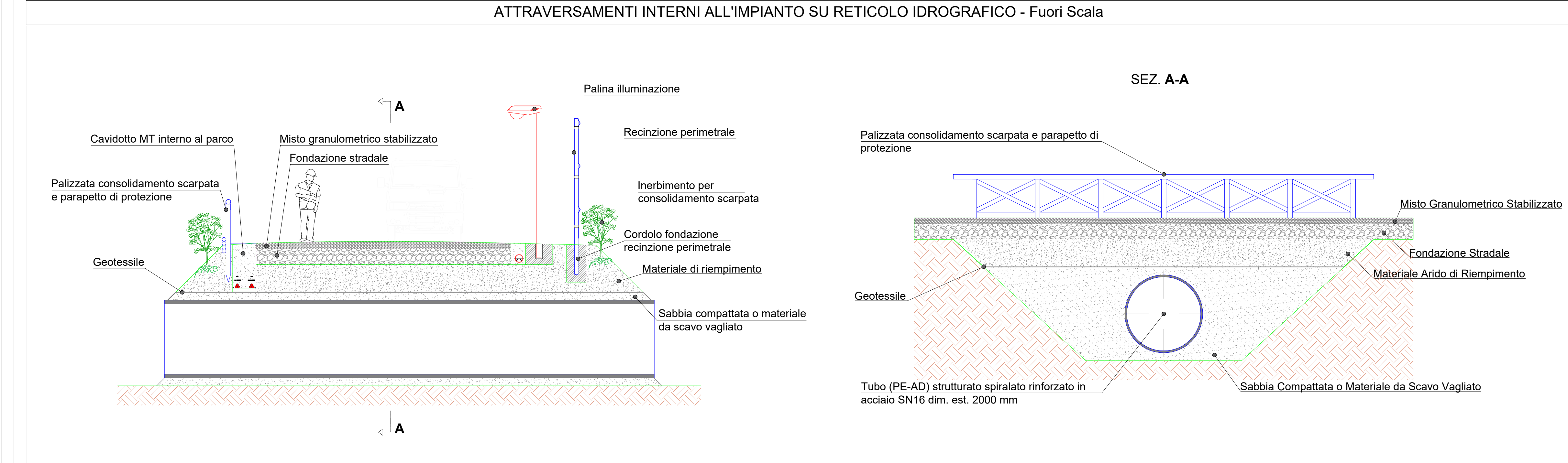
ATTRAVERSAMENTI INTERNI ALL'IMPIANTO SU RETICOLO IDROGRAFICO - Fuori Scala
