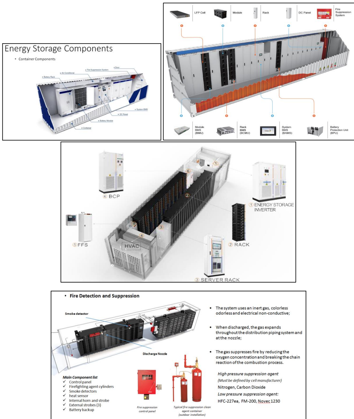
Fig. Strutture dei containers
