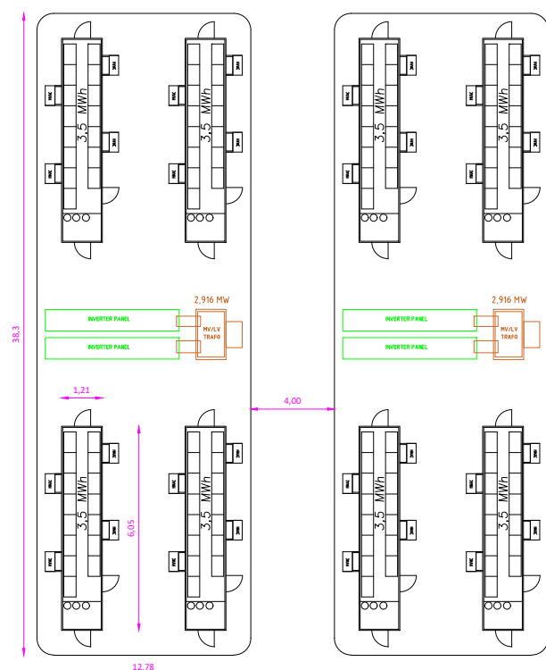
PARTICOLARE ACCUMULO scala 1.200
