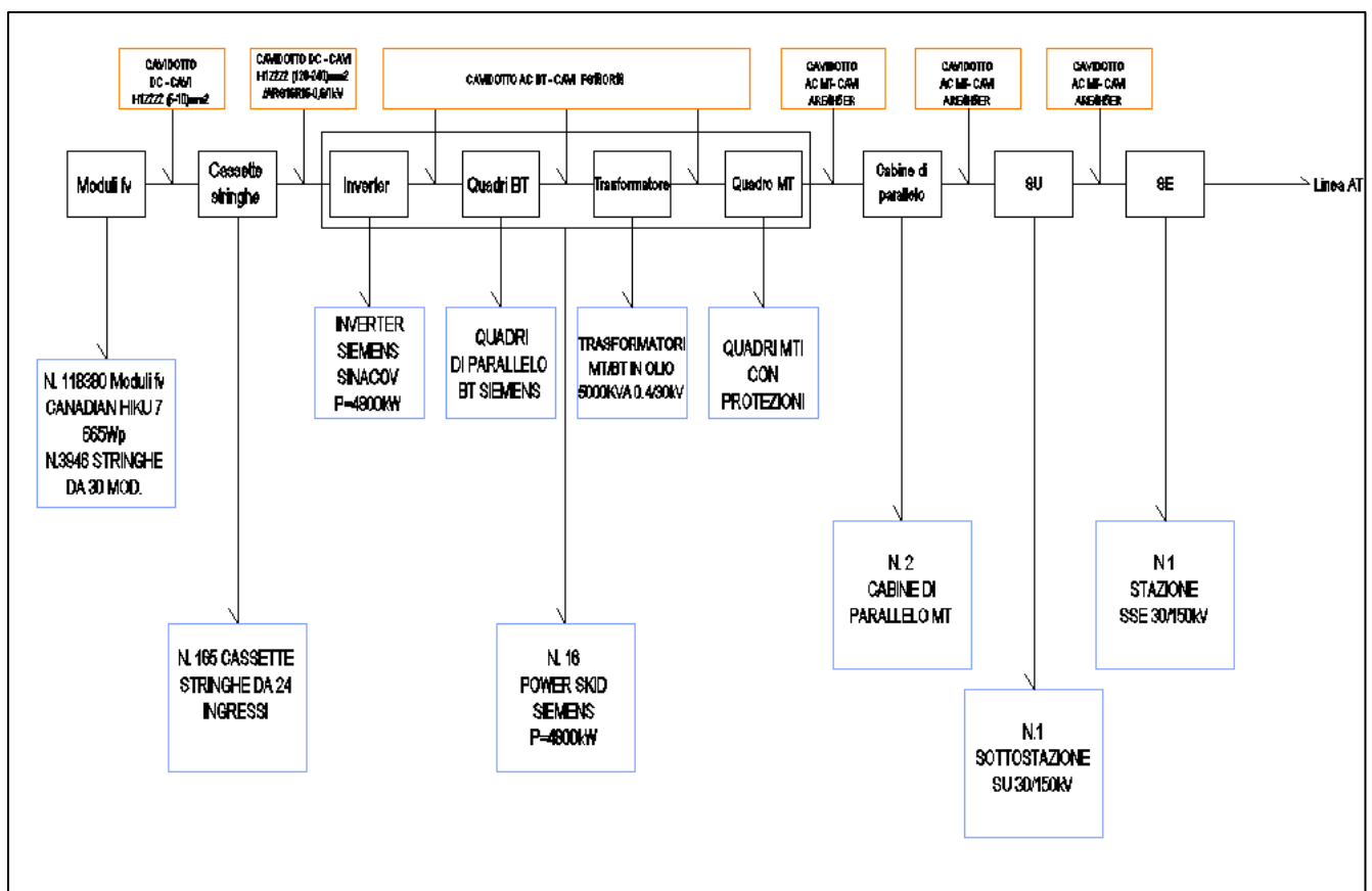
Figura 4 - Schema a blocchi impianto
