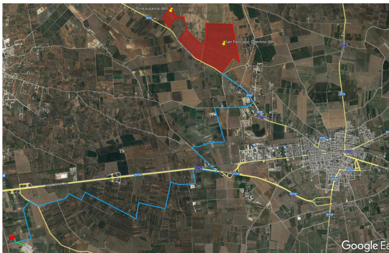
Figura 5 - Cavidotto MT da impianto a SU - SE Terna
