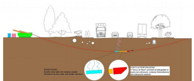
fase 1: REALIZZAZIONE FORO PILOTA CON CONTROLLO ALTIMETRICO
