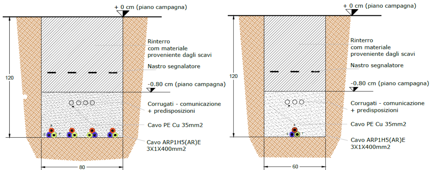
Fig. 4.4 Sezioni tipo scavo su terreno per cavidotto interno al campo di collegamento MT entra-esce tra Power Skid
