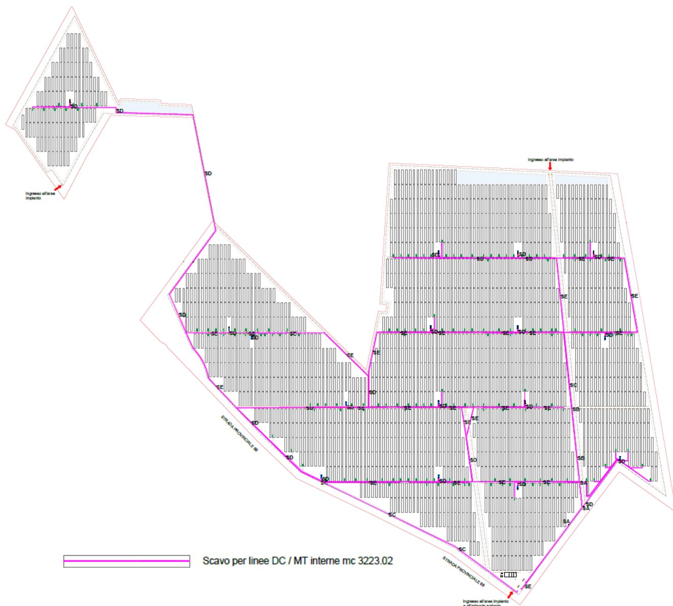
Fig. 4.3 Individuazione aree di scavo per le reti elettriche
