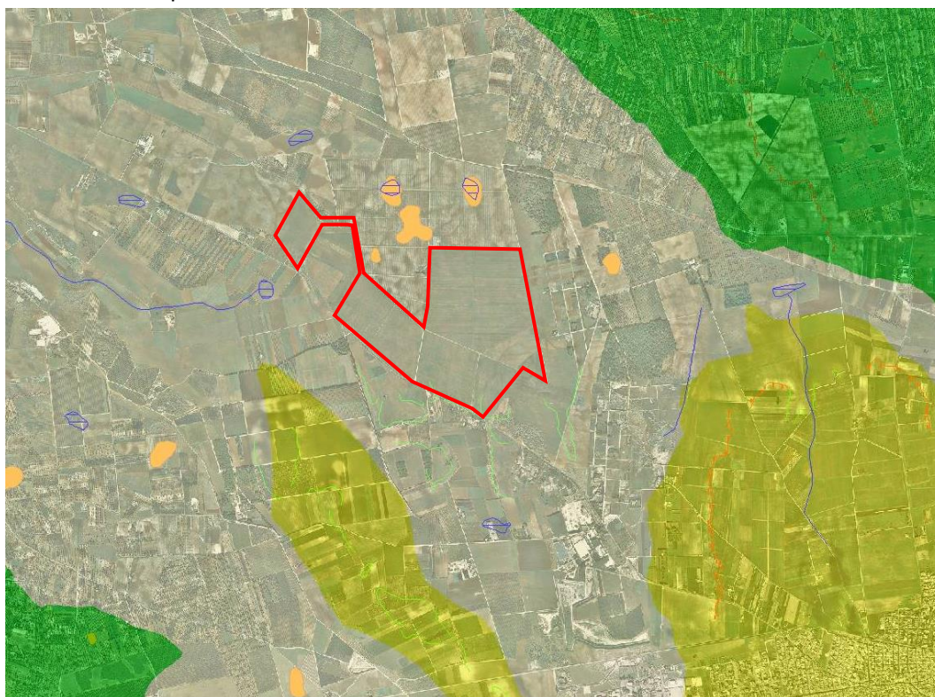
Fig. 3.3 Stralcio dell'area di intervento su Carta Idrogeomorfologica dell'AdB Puglia
