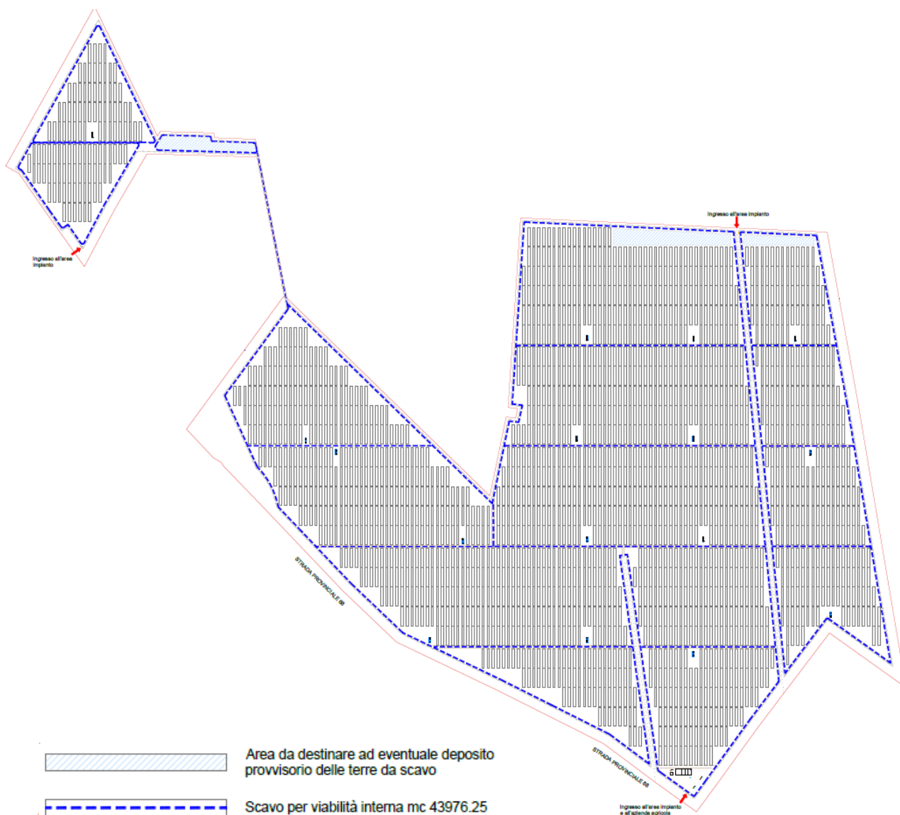
Fig. 4.2 Individuazione aree di scavo per la viabilità di campo
