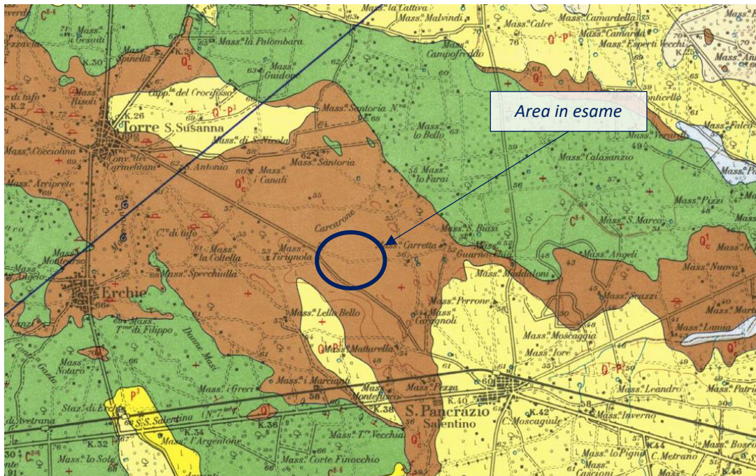
Fig. 3.2 Stralcio Foglio 203 della Carta geologica con ubicazione dell'area d'intervento
