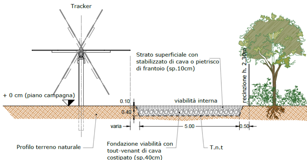
Fig. 4.1 Particolare di posizionamento tracker e scavo per viabilità
