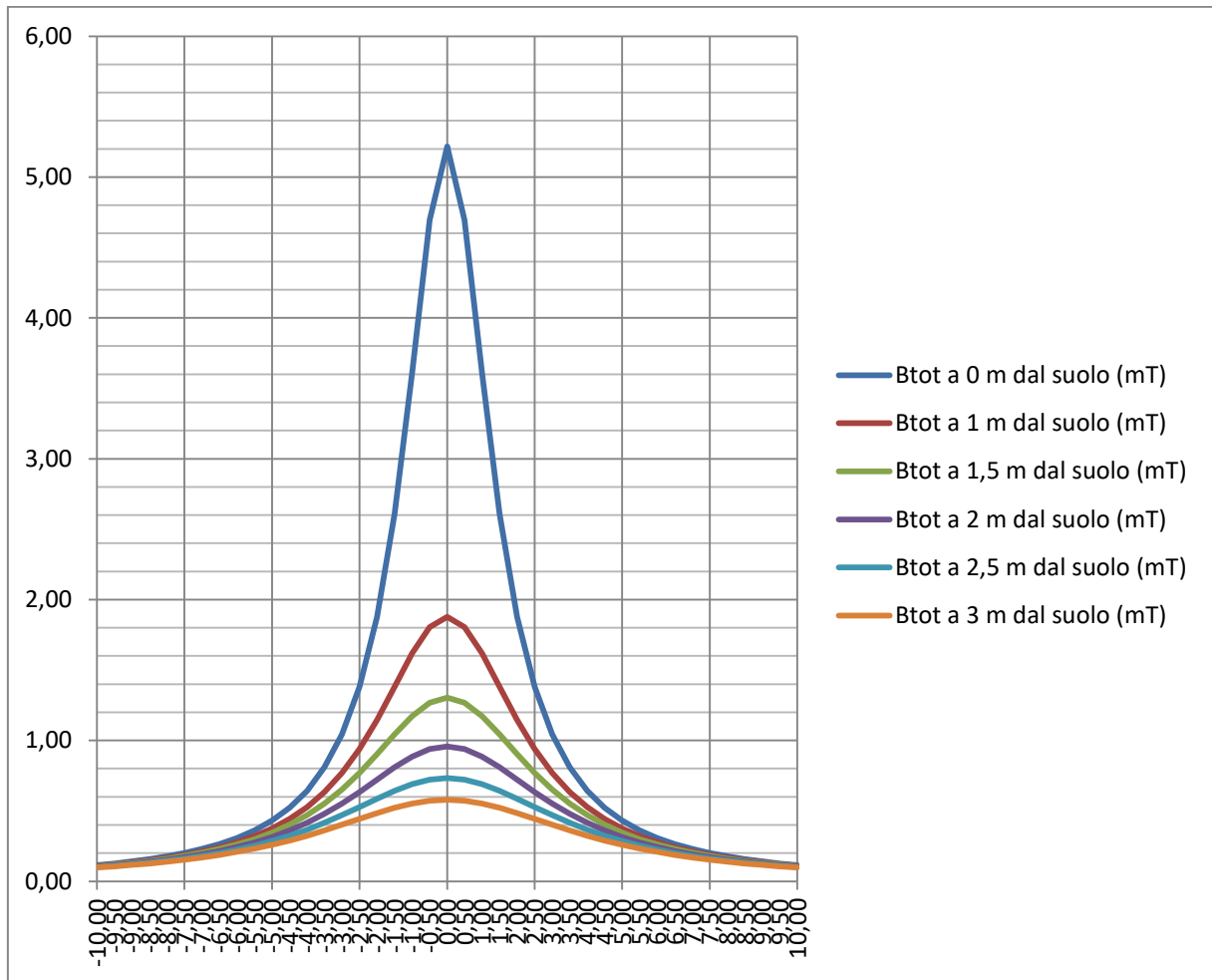
Grafico del campo di induzione magnetica per diverse distanze dall'asse dei cavidotti e altezze dal suolo Cavidotto esterno AT
